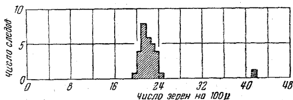
Рис. 3. Гистограмма, показывающая распределение значений средней плотности зёрен в следах частиц с малой удельной ионизацией.
