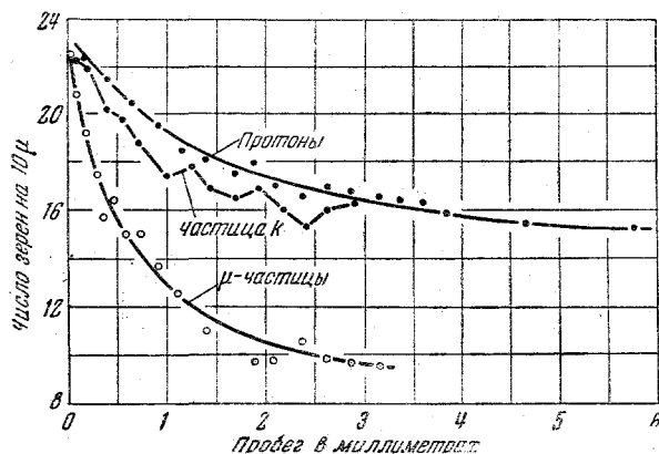
Рис. 10. Зависимости плотность зёрен — пробег для частицы k , протонов и \mu -частиц.
