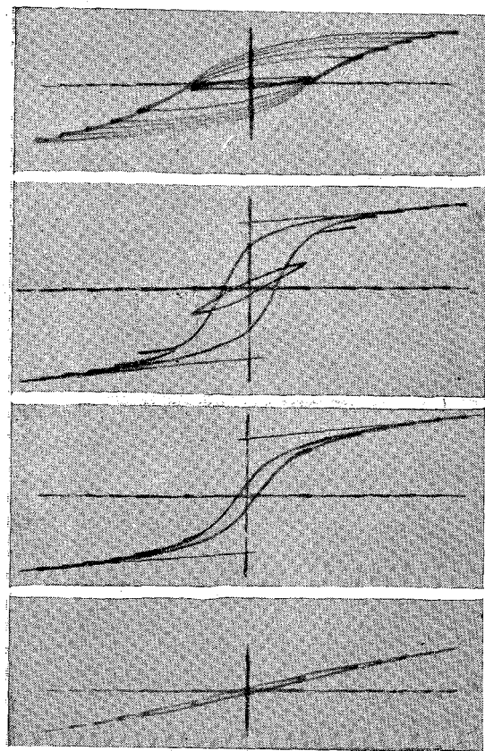
Рис. 7. Осциллограммы петель гистерезиса титаната бария при температурах -183^\circ\text{C} , 26,8^\circ\text{C} , 73,8^\circ\text{C} и 115,5^\circ\text{C} и напряжённости поля E = 25 \text{ кВ/см} .
