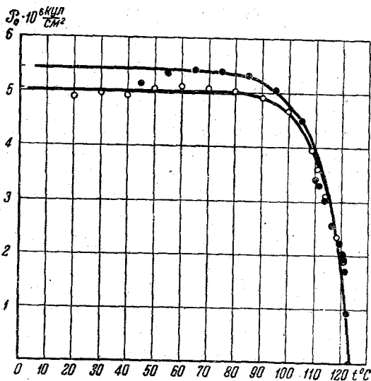
Рис. 9. Температурная зависимость спонтанной поляризации поликристаллических образцов титаната бария.
