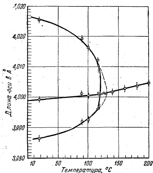
Рис. 1. Изменение длин осей и кубического корня из объема элементарной ячейки в зависимости от температуры.
