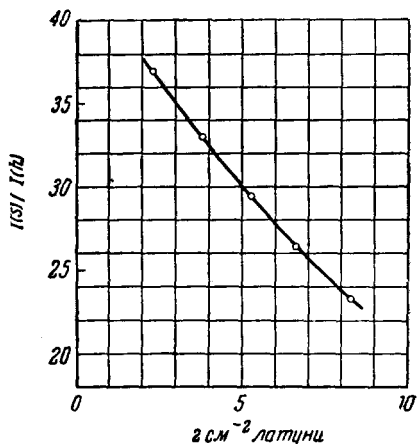
Рис. 1. Кривая поглощения «мягких» частиц космических лучей в латуни. По оси абсцисс отложен минимальный пробег мягких частиц, определяемый толщиной стенок счётчика. По оси ординат отложено отношение интенсивности мягкой компоненты к жёсткой на уровне моря.
