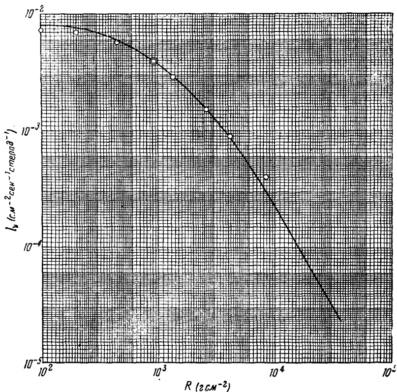
Рис. 5. Интегральный спектр пробегов мезонов на уровне моря. Пробег измеряется в \text{г см}^{-2} воздуха. Кружками показаны результаты измерений спектра импульсов W^7 , нормированные при 920 \text{ г см}^{-2} (двойной круг).
