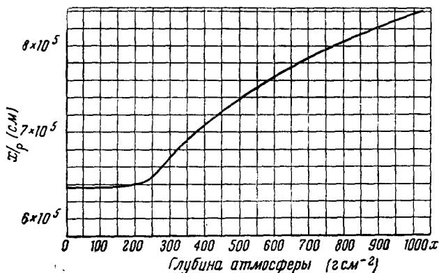
Рис. 21. x/r в функции x в стандартной атмосфере; x — глубина атмосферы, \rho — плотность воздуха.
