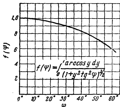
Рис. 26. График функции f(\psi) . Величина \operatorname{tg} \psi f(\psi)/\pi представляет относительное число вторичных частиц, удаляющихся от земли под углом \psi с вертикалью, в предположении, что эти частицы образуются первичной компонентой, изотропно распределённой в верхней полушфере.
