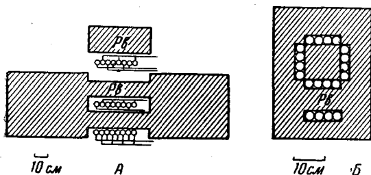
Рис. 11. Две установки для изучения жёстких ливней. А 13 ; совпадения регистрировались только в том случае, если по крайней мере в одном из счётчиков каждой из семи групп, показанных на рисунке, произошёл разряд. Б 16 ; совпадения регистрировались только в том случае, если по крайней мере в двух счётчиках каждой из трёх горизонтальных групп произошёл разряд. (Показанные на рисунке две вертикальные группы предназначались для получения дополнительной информации о структуре ливней.)
