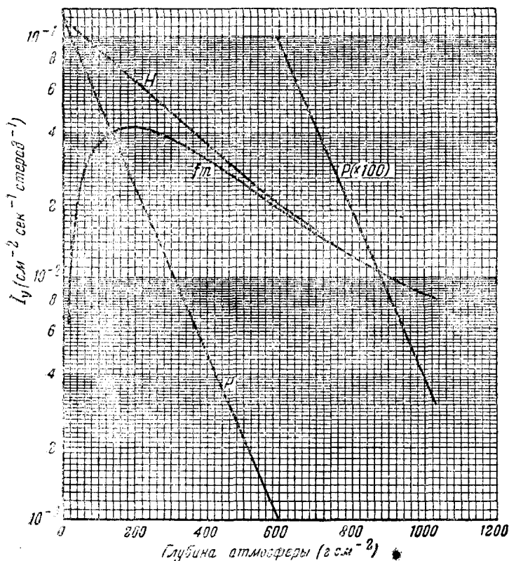
Рис. 16. Анализ жёсткой компоненты. Кривая f\pi показывает вертикальную интенсивность мезонов с пробегом, большим чем 167 \text{ г см}^{-2} свинца («быстрые мезоны»). Кривая P показывает вклад N -компоненты (протоны большой энергии) в измеренную интенсивность жёсткой компоненты, но не даёт абсолютного значения вертикальной интенсивности N -компоненты.
