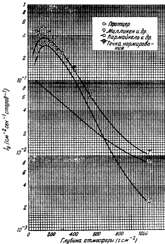
Рис. 2. Вертикальная интенсивность жёсткой компоненты (H), мягкой компоненты (S) и всей ионизующей компоненты (T), как функция глубины атмосферы на геомагнитных широтах, больших 45^\circ . Минимальный пробег мягких частиц равен 5 \text{ г см}^{-2} латуни.
