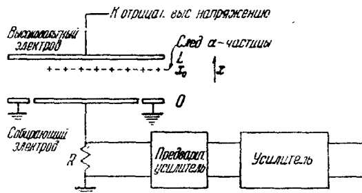
Рис. 1. Типичное устройство плоского ионизационного счётчика. Значки плюс и минус обозначают ионы вдоль следа \alpha -частицы.
