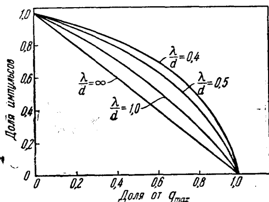
Рис. 18. Интегральная кривая распределения величин импульсов, на которой доля импульсов, больших чем определённая доля от q_{\max} , представлена в функции q_{\max} .
