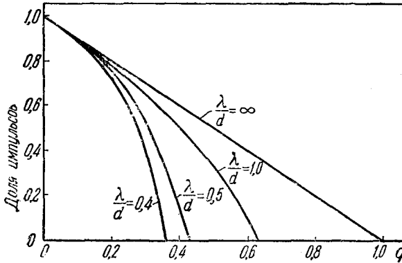
Рис. 17. Интегральная кривая распределения величин импульсов для тех же условий, что и на рис. 16. Доля импульсов, больших чем данное q , представлена как функция q .
