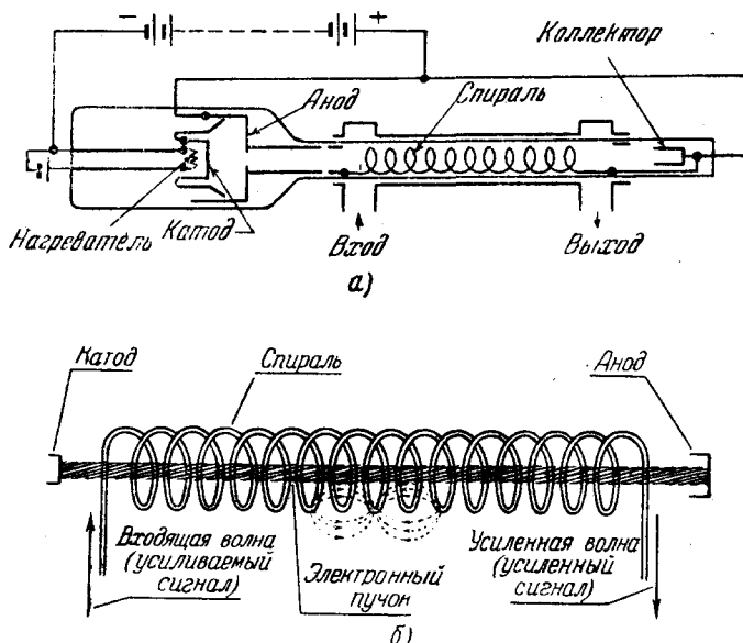
Рис. 3. Схема усилителя с бегущей волной. На рис. (а) показаны подогревный катод, ускоряющий электрод, спираль, замедляющая волну, коллектор электронов. Подача сигнала и его вывод осуществляются с помощью волноводов. На рисунке (б) даны спираль и электронный пучок в увеличенном масштабе.
