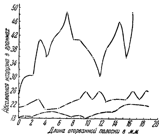
Рис. 10. Колебания нагрузки при отрыве с постоянной скоростью; нижняя кривая — нитроцеллюлоза-стекло; средняя — каучук-стекло; верхняя — гуттаперча-стекло.
