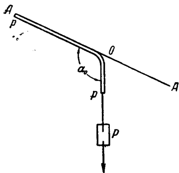
Рис. 1. Схема метода для измерения адгезии эластичных плёнок.
