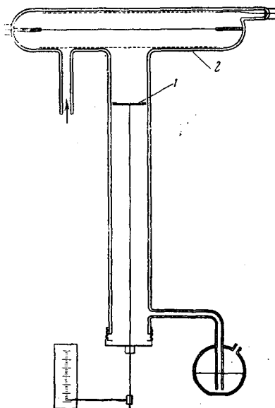
Рис. 1. Схема счётчика для обнаружения мягкого излучения:
