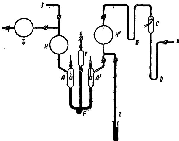
Рис. 10. Схема установки для обогащения водорода и дейтерия тритием путём электролиза: A , A' — сосудов для электролиза; B , C , D — осушка и выжигание газа; E — ловушка с водой, содержащей тритий; G , H — сосуды для сбора газа.
