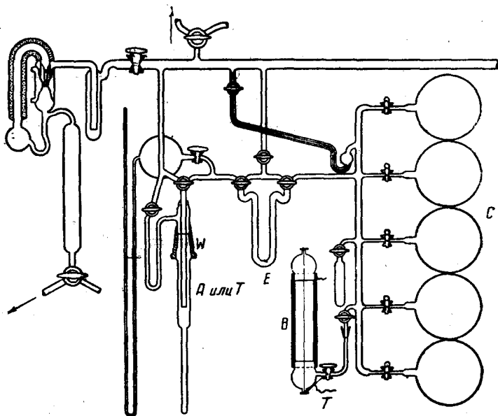
Рис. 12. Схема установки для определения трития, содержащегося в растворенной в бензоле воде: A — сосуд с образцом, содержащим тритий; B — счётчик; C — колбы; E — U-образная трубка с \text{CaO} .
