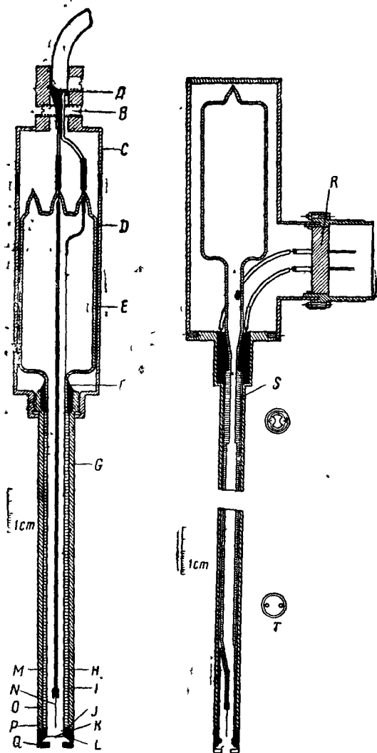
Рис. 8. Схема счетчика со свинцовым окошком: K — окошко; N — нить; M — катод; G — защитная рубашка; R — вводы.
