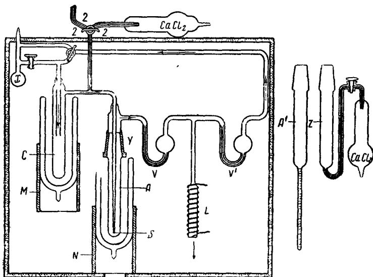
Рис. 11. Схема установки для насыщения растворителя малым количеством воды: А — сосуд для насыщения; А' — сосуд с калиброванным капилляром для переноса образца; S — капилляр для пропускания воздуха, насыщенного парами воды.
