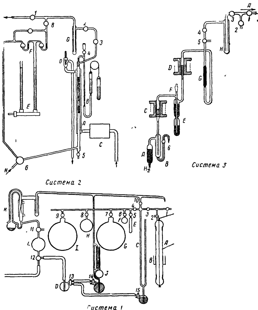
Рис. 6. Схема установки для определения равновесия системы вода—триций: Система 1. A — счётчик Гейгера-Мюллера; B — ванночка со стандартным раствором соли урана; C — манометр; D — ловушка; E , F , G , H , I — сосуды для хранения газов, воды и спирта; J — манометр Мак-Леода; K — ртутный насос, 1 — 15 — краны. Система 2. A — трубка с катализатором; B — приспособление для впуска воды в трубку A ; C — циркуляционный насос; E — насос, 1 — 8 — краны. Система 3. A — B — ловушки; E — ловушка с водой, содержащей триций G — трубка с катализатором, 1 — 6 — краны.
