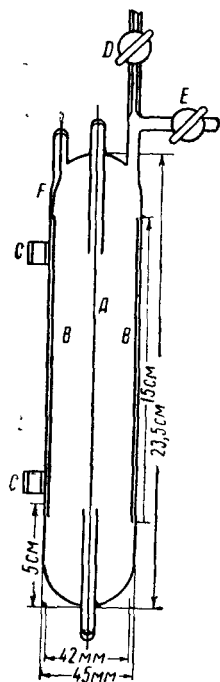
Рис. 9. Схема счётчика, работающего при введении активного вещества вместе со счётным газом: А — нить; В — катод; С — ванночки со стандартным раствором; D, E — краны.
