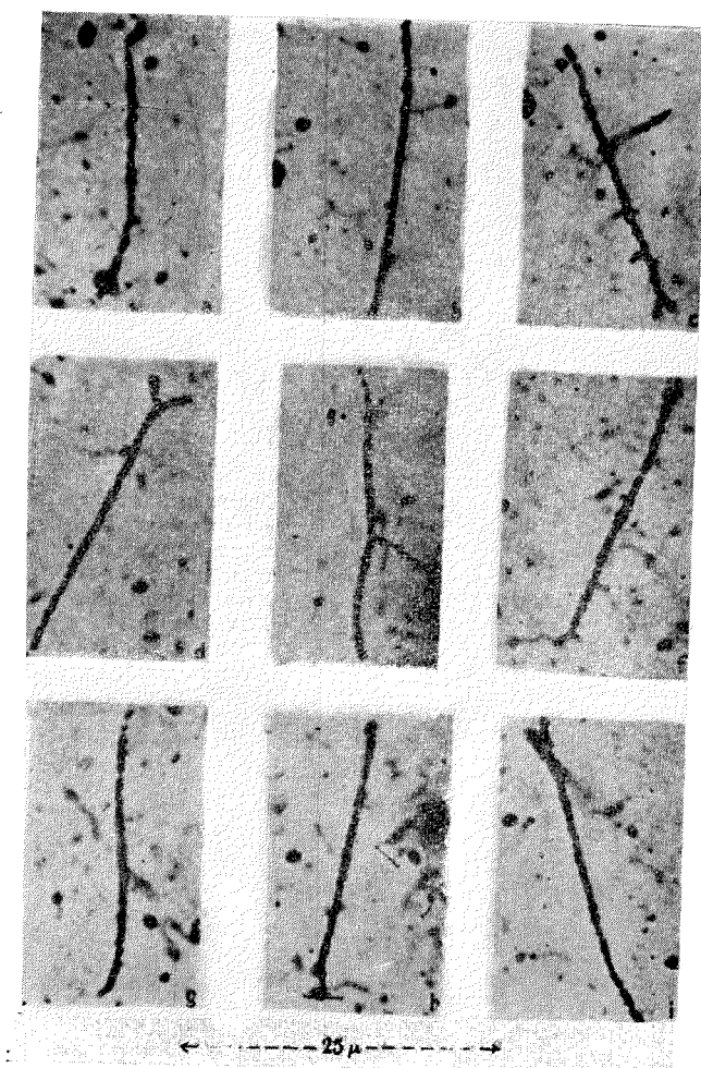
Следы деления U^{235}
