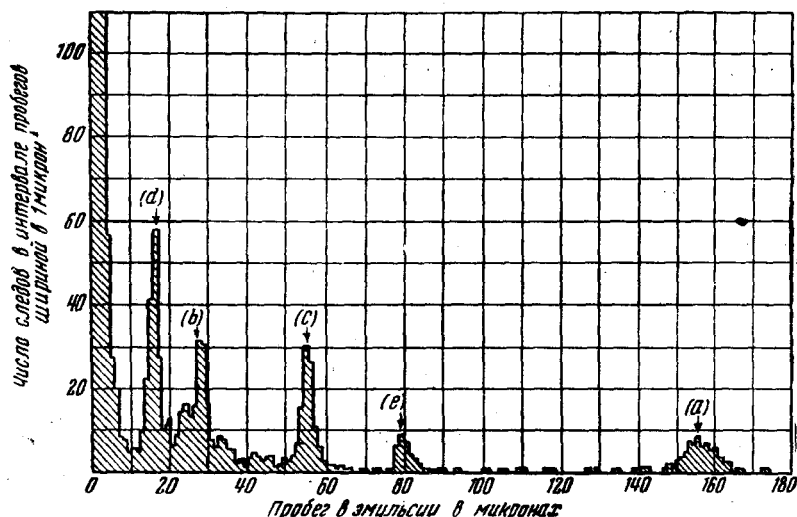
Рис. 13. Распределение по пробегам следов, получающихся при расщеплении бериллия дейтронами с энергией 900 KeV
