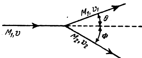
Рис. 12. Диаграмма импульсов.
