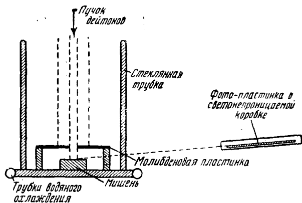
Рис. 15. Схема установки для исследования распределения по энергиям нейтронов, возникающих при расщеплении лёгких элементов быстрыми дейтонами.
