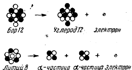
Рис. 10. Два примера изменения состава ядер при бета-распаде.
