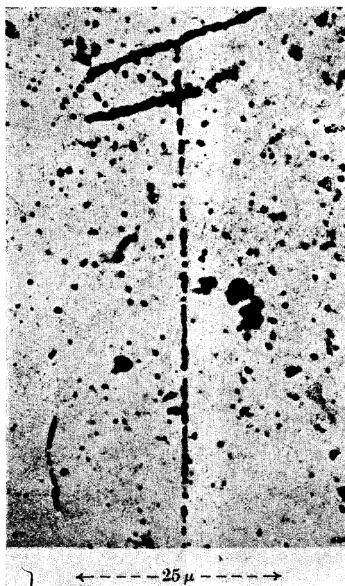
Следы деления ядра на три части, из которых одна является \alpha -частицей
