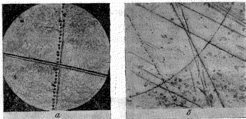
Рис. 11. Микроповреждения латуни после кратковременной кавитации в воде, имеющие линейчатый характер; а —увеличено в 400 раз, б —увеличено в 1200 раз.
