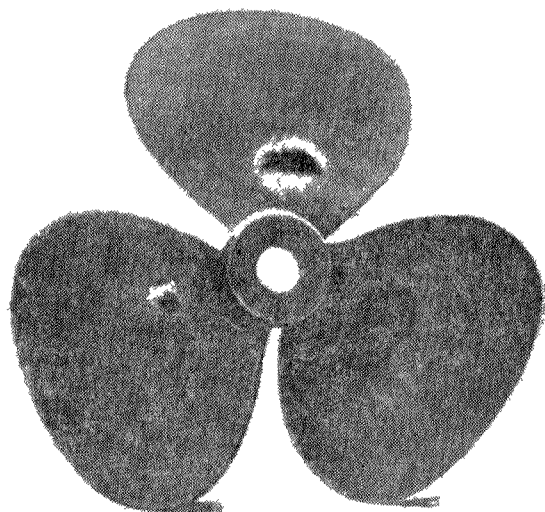
Рис. 1. Кавитационные повреждения лопастей гребного винта.
