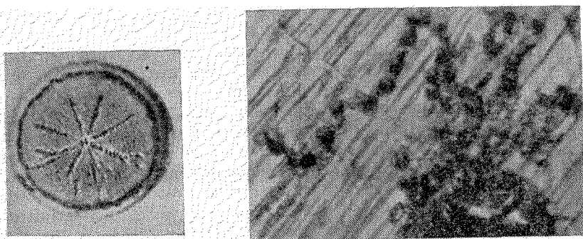
Рис. 11. Микроповреждения латуни после кратковременной кавитации в воде, имеющие линейчатый характер; а —увеличено в 400 раз, б —увеличено в 1200 раз.
