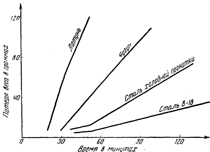
Рис. 4. Потеря веса образцов, сделанных из различных материалов, вызванная кавитационными повреждениями, в функции времени кавитации.
