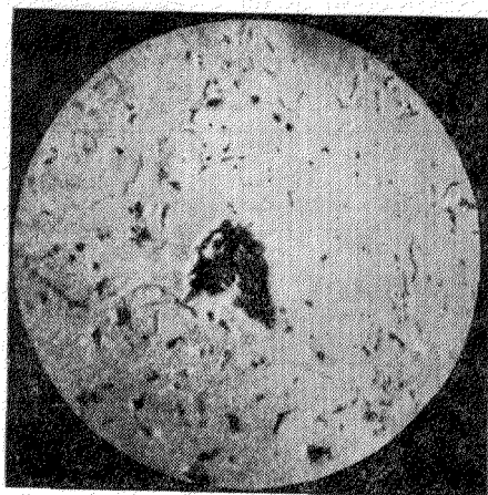
Рис. 20. Кавитационные повреждения стеклянной пластинки (увеличено, примерно, в 200 раз).
