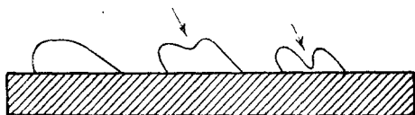
Рис. 19. Последовательные изменения формы кавитационного пузырька при его сжатии.
