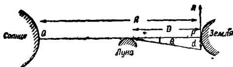
Рис. 4. Дифракция на лунном крае.
