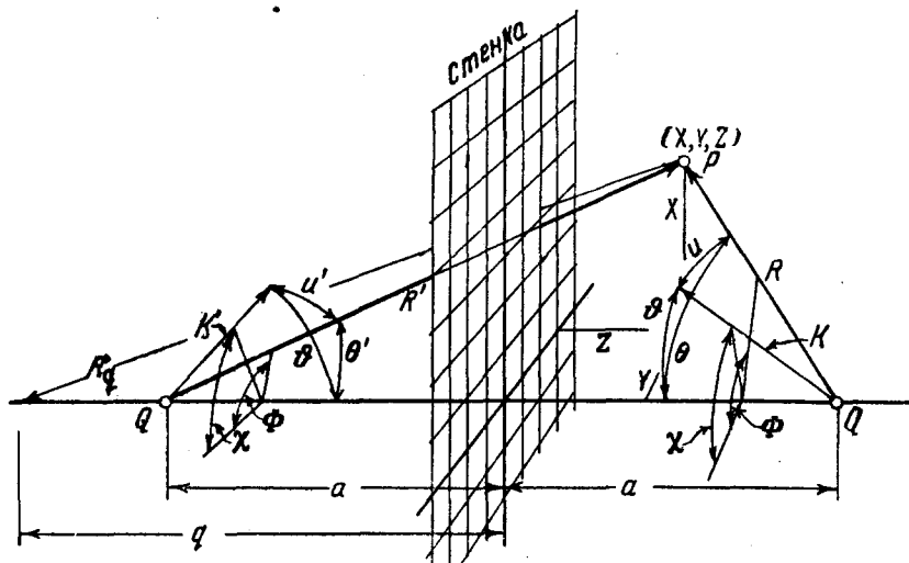
Рис. 31. Обозначения углов и расстояний, принятые при расчёте отражения сферической волны от поглощающей стенки.
