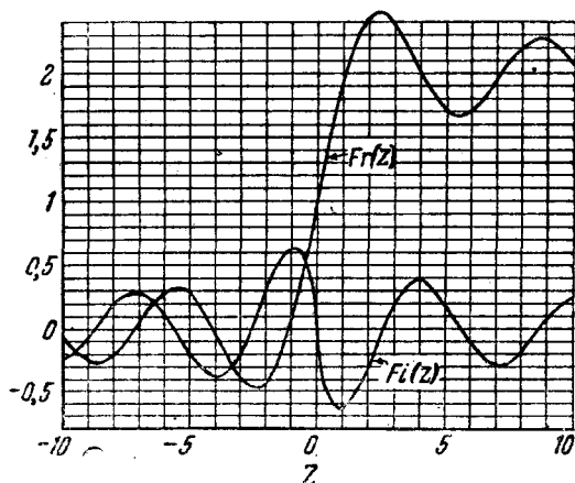
Рис. 32. Дифракционные функции, входящие в расчёт краевых поправок.
