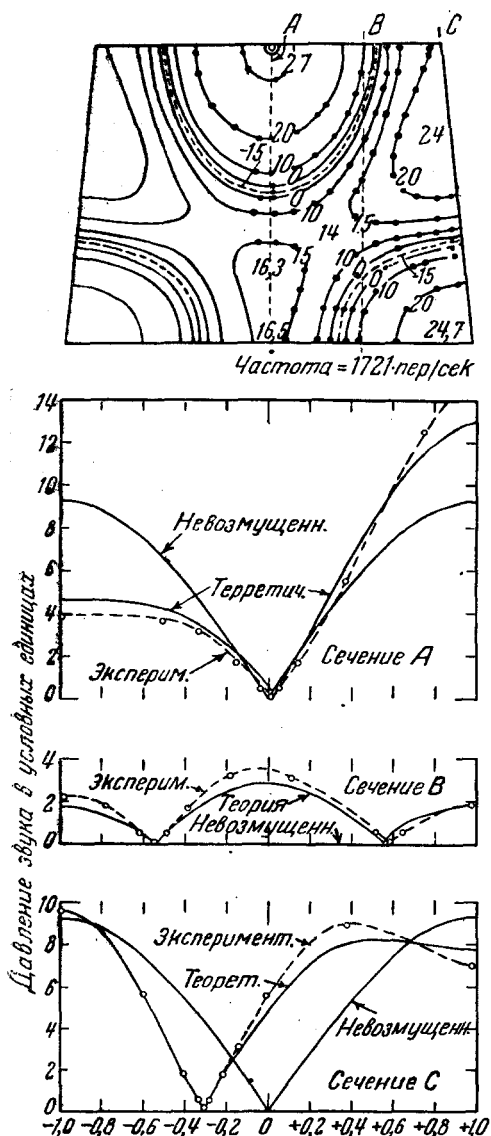
Рис. 29. Распределение давления в стоячей волне по измерениям в трапециoidalном помещении. Нижние кривые сопоставляют экспериментальные результаты (пунктирные линии) с результатами подсчёта возмущений второго порядка (сплошные линии, вычисленные теоретически) В10.
