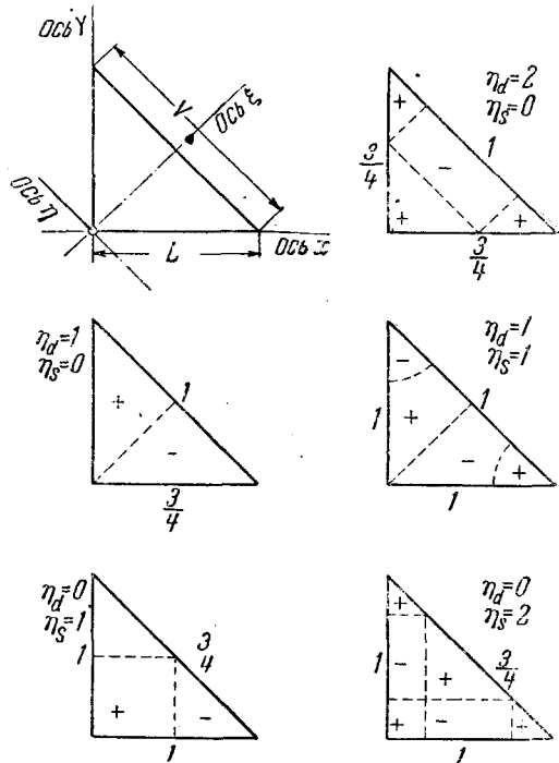
Рис. 27. Расположение узловых фигур давления в треугольном помещении и значения коэффициента типа колебаний e_N . Целые числа — n_d и n_s ; соответствующие значения e_N надписаны около каждой стенки.
