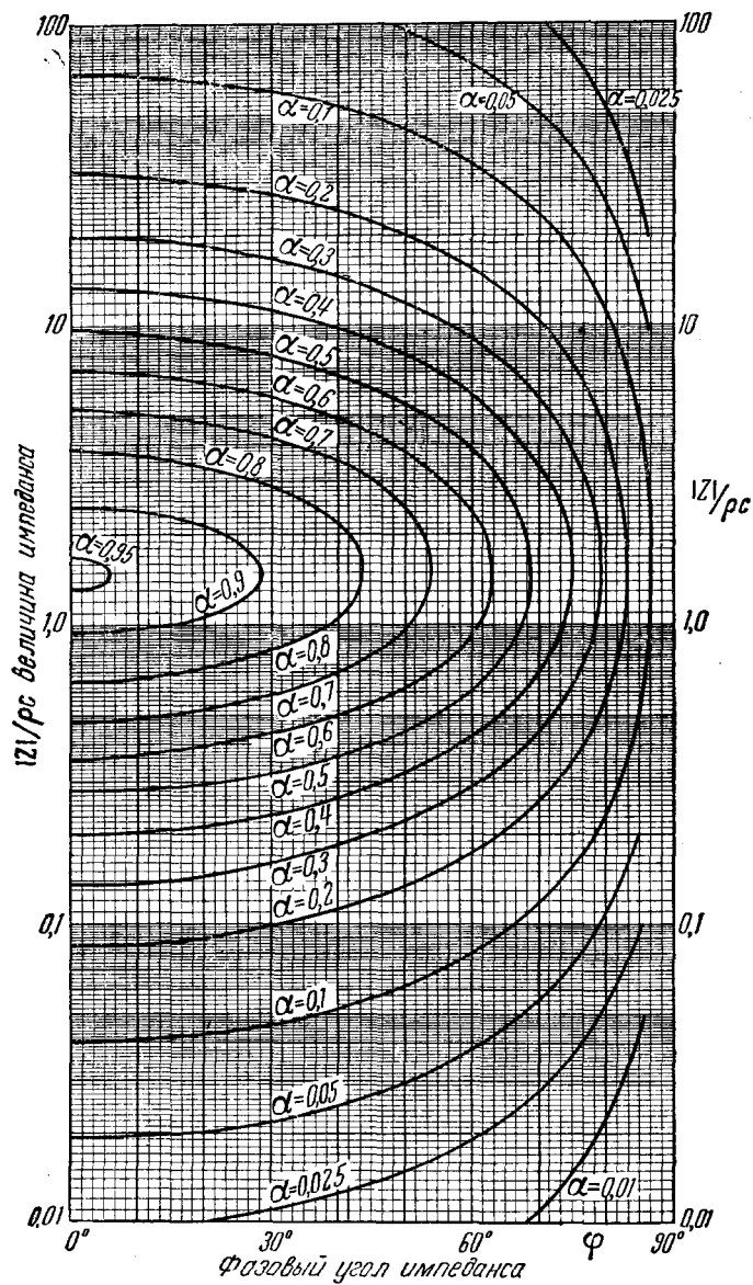
Рис. 30. Сэбинский коэффициент поглощения \alpha стат в функции от модуля и аргумента импеданса стенки. Диаграмма относится к случаям, когда имеет место эргодический звуковой процесс.
