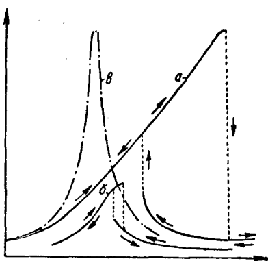
Рис. 4. Кривая феррорезонанса.
