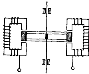
Рис. 2. Конструкция, обеспечивающая периодическое изменение самоиндукции.
