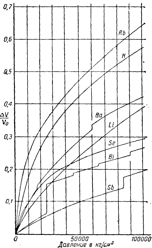
Рис. 3. Уменьшение объема нескольких элементов до 100\,000\text{ кг/см}^2 . Изломы в некоторых кривых указывают на наличие полиморфных превращений.
