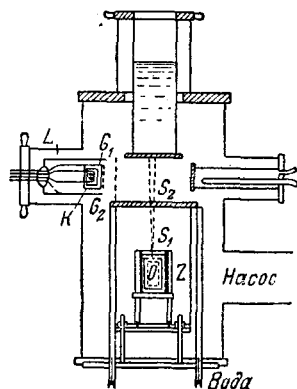
Рис. 3. Аппарат Пауля для веществ с высокой точкой плавления.
