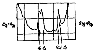
Рис. 5. Интерференционные картины линий натрия.
