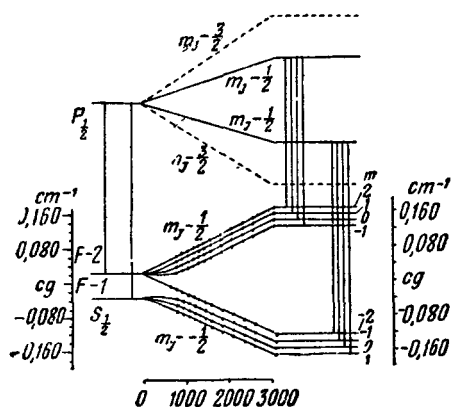
Рис. 4. Диаграмма термов эффекта Зеемана линии натрия 3^2S_{1/2} - 3^2P_{1/2} .
