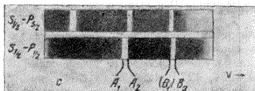
Рис. 5. Интерференционные картины линий натрия.
