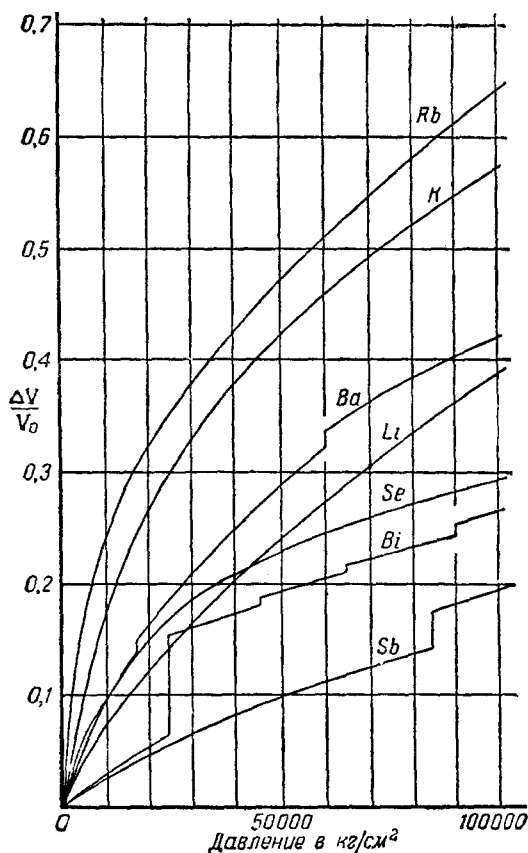
Рис. 15. Объемная сжимаемость элементов при давлении в 100\,000\text{ кг/см}^2 . Скачки на кривых соответствуют полиморфным превращениям.
