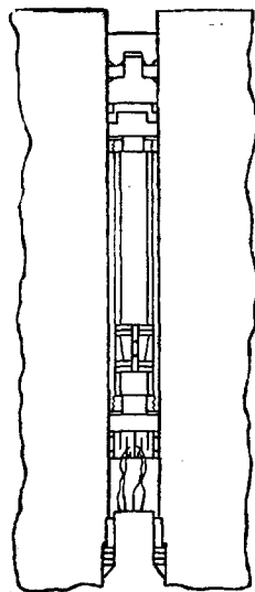
Рис. 13. Прибор малого размера, погружённый в жидкость большого прибора для давлений в 25\,000\text{ кг/см}^2 и выше, позволяющий получить давление в 100\,000\text{ кг/см}^2 . Испытуемое вещество сдавливается с двух сторон двумя поршнями из карболоя. Цилиндр малого прибора изготовлен из карболоя и охвачен стальным кольцом.
