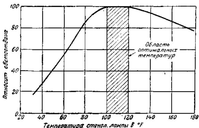
Рис. 15. Светотдача, как функция температуры стенок люминесцентной лампы.
