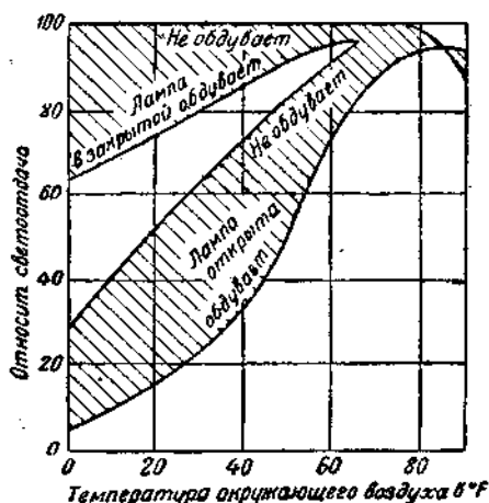
Рис. 28. Светоотдача люминесцирующей лампы в зависимости от температуры окружающего воздуха. Обдувание вызывает снижение температуры стенок. Наоборот, заключение лампы в герметичную арматуру повышает температуру стенок.
