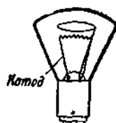
Рис. 30. Ультрафиолетовая люминесцентная лампа постоянного тока 24 В.
