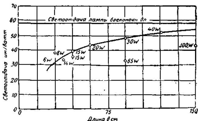
Рис. 14. Светотдача люминесцентной лампы, как функция её длины.
