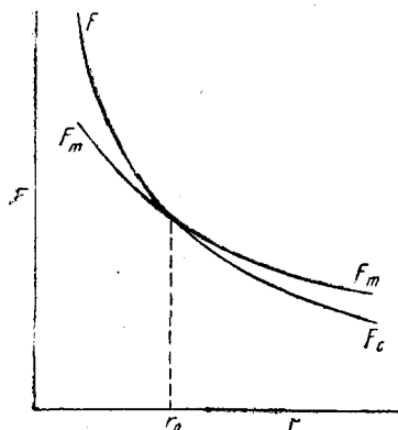
Рис. 2. Сила F_c \left[ = \frac{mv^2}{r} \right] представляет собой центростремительную силу, необходимую для удержания электрона на окружности радиуса r ; F_m \left[ = \frac{e}{c} H v \right] — сила, с которой магнитное поле действует на электрон в действительности. Равновесная орбита соответствует абсциссе r = r_0
