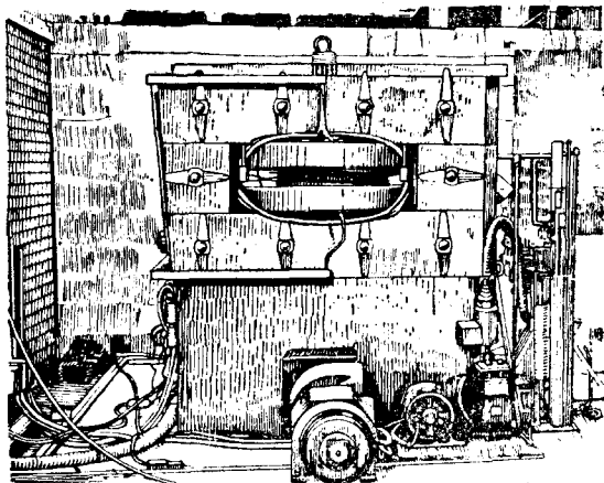
Рис. 3. Новый бетатрон, дающий электроны с энергиями до 20 \cdot 10^6 eV. Светлое пятнышко на камере между полюсами электромагнита обязано своим происхождением инжектору
