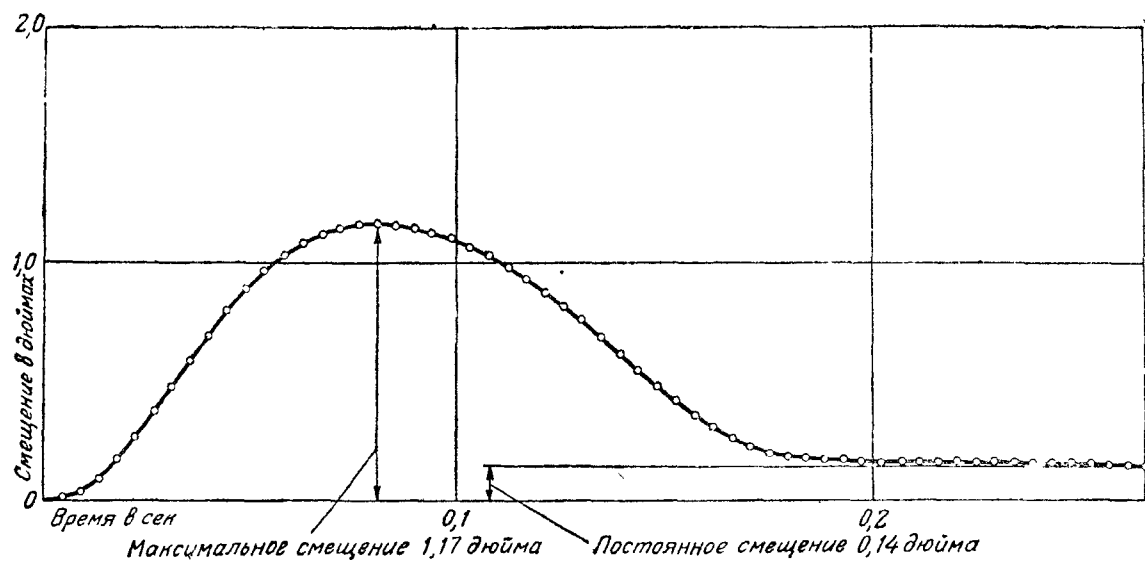
Рис. 3. Запись смещения.
