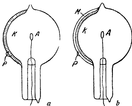
Рис. 4 Схема строения Sb-Cs-катодов: а — катод без подкладки, б — катод на подкладке
