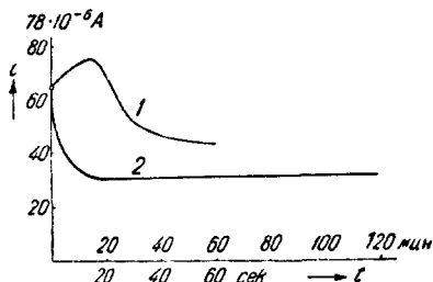
Рис. 9. Утомление Sb-Cs-фотоэлементов на больших освещенностях ( \sim 4 \cdot 10^4 lx). Нижний масштаб оси времени — для кривой 1. По оси ординат отложен фототок при неизменном освещении
