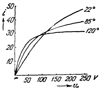
Рис. 6. Изменение хода вольтамперных кривых фотоэлемента без подкладки в зависимости от температуры (по оси координат отложен фототок в относительных единицах)
