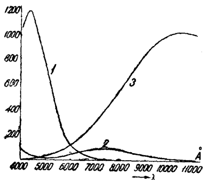
Рис. 3. Распределение чувствительности по спектру для Sb-Cs (1) и Cs-O-Ag (2) фотозlementов в одном масштабе для фототока и (3) распределение энергии в спектре лампы накаливания
