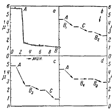
Рис. 3. Влияние кислорода на трение чистых металлов
