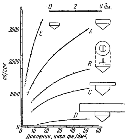
Рис. 5. Кривые A, B, C и D получены с неподвижным статором и роторами, изображенными справа от кривых. Кривая E снята с подвижно укрепленным статором (Бимс)
