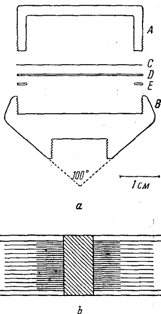
Рис. 7. Разрез ротора закрытого типа (а) и вкладыш к нему (б)
