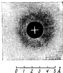
Рис. 1. Распределение электронов в атоме натрия по волново-механической теории
