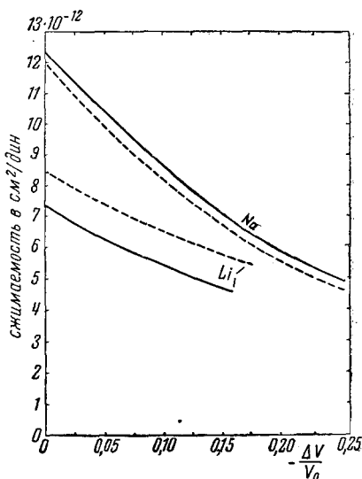
Рис. 6. Сжимаемость в функции сжатия. Сплошные кривые — экспериментальные, пунктирные — теоретические
