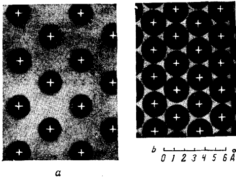
Рис. 10. Распределения электронов:
