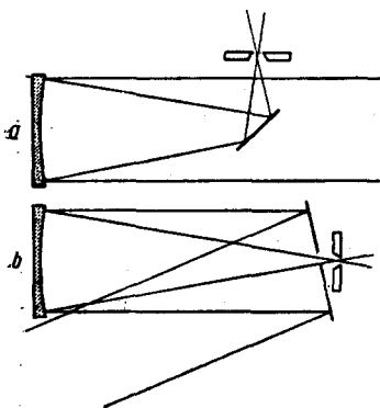
Рис. 4. Устройства вспомогательных зеркал для достижения перпендикулярного падения на вогнутые зеркала
