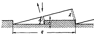
Рис. 28. Возникновение спектра первого порядка у ламинарной решетки
