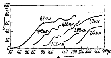
Рис. 24. Пропускание плавленого кварца
