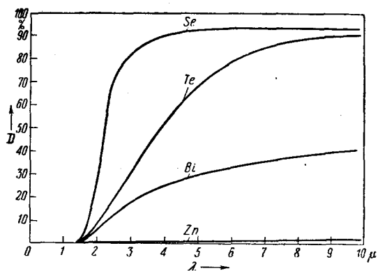
Рис. 2. Пропускание Se-, Te-, Bi- и Zn-черни в зависимости от длины волны. Толщина слоев выбрана так, что пропускание начинается при одинаковых длинах волн
