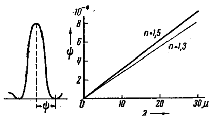
Рис. 10. Минимальная ширина \phi спектральной линии для призмы 60^\circ с длиной основания 5 см. Зависимость ее от длины волны \lambda и от показателя преломления n
