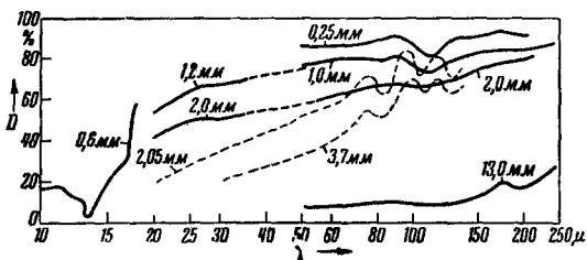
Рис. 25. Пропускание парафина: — точка плавления 68-72^{\circ}\text{C} , ---- точка плавления 42-44^{\circ}\text{C}
