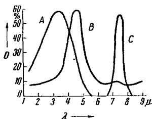
Рис. 12а. Пропускание фильтра Христиансена из порошкообразного кварца: А — в \text{CS}_2 + \text{CCl}_4 (1:1), В — в \text{CCl}_4 , С — в воздухе
