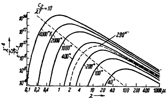
Рис. 1. Изотермы, отвечающие закону излучения Планка в дважды логарифмическом представлении
