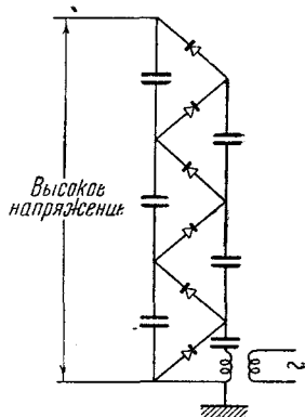
Рис. 11. Схема Грейнахера
