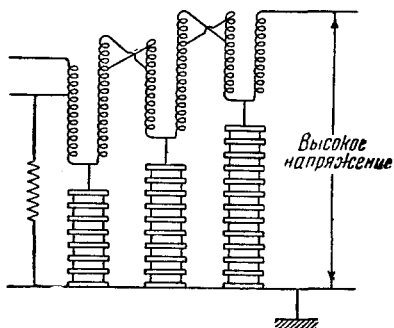
Рис. 10. Схема каскадного трансформатора
