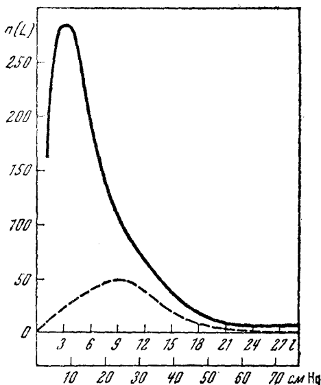
Рис. 4. Общая интенсивность космических лучей, идущих в вертикальном направлении, как функция высоты в атмосфере по Регенеру—Пфоперу. Пунктиром дана теоретическая кривая для экватора.
