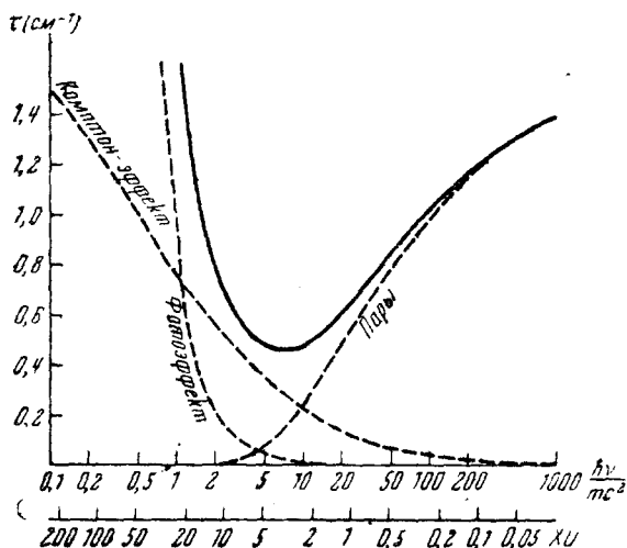
Рис. 2. Коэффициент поглощения \gamma -лучей в свинце как функция энергии фотона в логарифмической шкале. Пунктиром нанесены доли, приносимые фотоэффектом, комптон-эффектом и образованием пар
