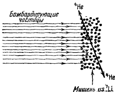
Рис. 17. Схема, иллюстрирующая превращение изотопа лития с массой 7 при протонной бомбардировке. На каждую сотню миллионов протонов с энергией в 200 000 В одно ядро лития превращается в два гелиевых ядра. Длина пробега возникающих \alpha -частиц около 8,4 см.
