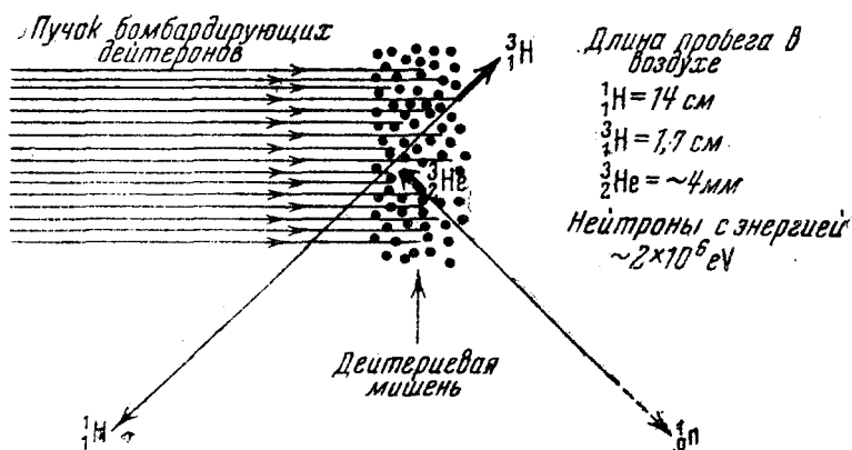
Рис. 20. Схема расщепления дейтерия при бомбардировке дейтонами. Около 2 млн. дейтронов с энергией 100 000 V бомбардирующих мишень из чистого дейтерия, производят одно превращение по какой-либо из двух указанных реакций.
