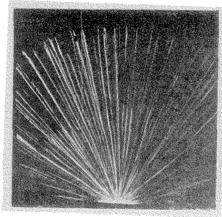
Рис. 3. Следы \alpha -частиц, испускаемых торием ( C + C' ), разделяющиеся на две группы с пробегами 8,6 см и 4,8 см в воздухе.
