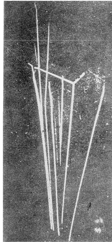
Рис. 9. Следы \alpha -частиц в кислороде. Один след на конце раздваивается в результате столкновения с ядром кислорода, причем короткая ветвь принадлежит отброшенному ядру кислорода, а более длинная — отклонившейся \alpha -частице. Измерения углов отклонения двух ветвей показали, что количество движения и энергия при данном столкновении сохраняются.
