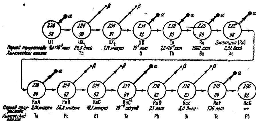
Рис. 1. Ряд превращений урана. Верхняя цифра в каждом кружке означает атомный вес, нижняя — порядковый номер элемента и заряд ядра. Длина жирной стрелы показывает относительную длину пробега \alpha -частиц.
