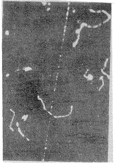
Рис. 4. Следы фотоэлектронов с пробегом около 1 см, образованных при абсорбции характеристического K -излучения серебра в воздухе (энергия около 21 000 V). Прямолинейный след принадлежит электрону с гораздо большей энергией и, вероятно, вызван космическими лучами.
