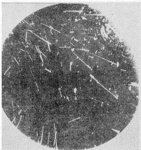
Рис. 11. Следы протонов отдачи, возникающие при обстреле метана нейтронами с энергией в 2,4 млн. V. Источник нейтронов помещался в S, где мишень из тяжелого водорода бомбардировалась ускоренными дейтронами
