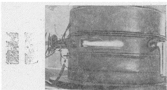
Рис. 5. Фотография 5\mu\text{A} -потока дейтронов с энергиями в 5,8 MeV (длина пробега в воздухе равна 25 см), выходящего из платинового окошка циклотрона.
