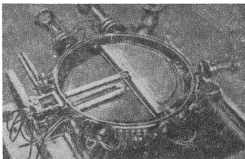
Рис. 3. Вид камеры циклотрона со снятой крышкой и удаленным дуантом (одним). В этом приборе ионы не удаляются полностью, но бомбардируют электроды на стенках камеры.
