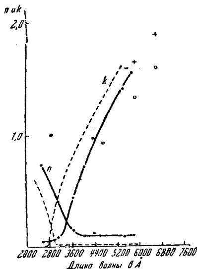
Рис. 4. Оптические постоянные калия: — данные Айвса и Бриггса, о — данные Денкен, 1-е зеркало, + — данные Денкен, 2-е зеркало, — — — вычислено по Кронгу
