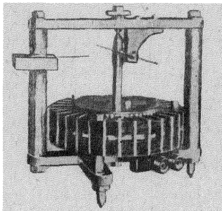
Рис. 20. Синхронный мотор
