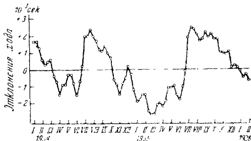
Рис. 37. Ход изменений между измеренными и вычисленными значениями \bar{G} для кварцевых часов III
