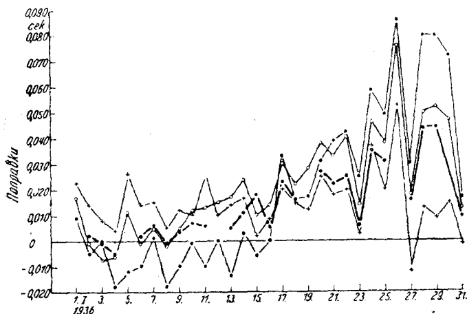
Рис. 5. Поправки к науэнскому сигналу времени, передаваемому в 13^h 01^m по данным Потсдама (ооо), Гамбурга (++++), Парижа (---), кварцевых часов III (—о—).
