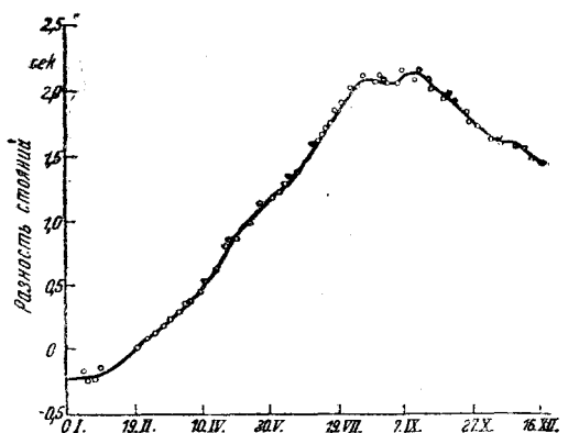
Рис. 10. Разности между измеренными и вычисленными стояниями часов Шортта № 11
