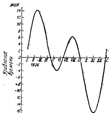
Рис. 1. Кривая уравнивания времени
