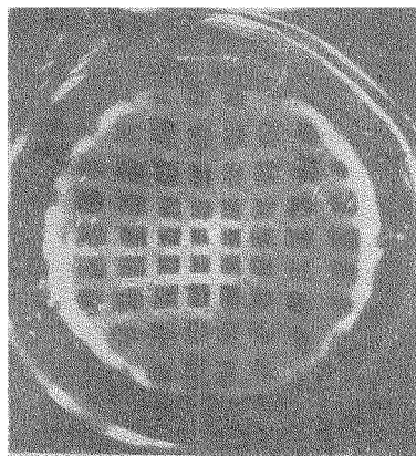
Рис. 13. Искажения изображения сетки при применении электрической электронной линзы (по Зворыкину и Мортону)
