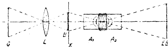
Рис. 1. Схема электроннооптического преобразователя изображений
