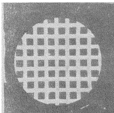
Рис. 14. Улучшение электронного изображения при применении искривленного катода (по Зворыкину и Мортону)
