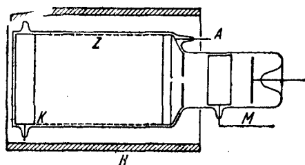
Рис. 6. Телевизионная трубка Фарнсворта
