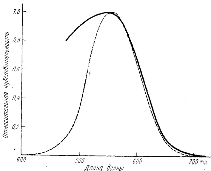
Рис. 8. Спектральная чувствительность селен-сернистых фотоэлементов
