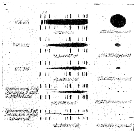
Рис. 9. Слева — спектры далеких туманностей; спектр сравнения принадлежит гелию
