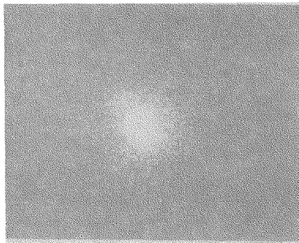
Рис. 4. Шарообразная звездная куча Мессье 13
