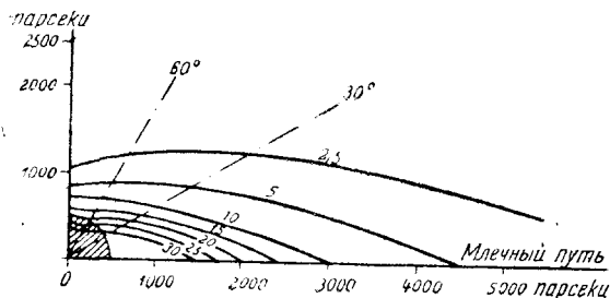
Рис. 2. Разрез местной звездной системы; ход кривых одинаковой частоты встречаемости звезд по Зеелигеру
