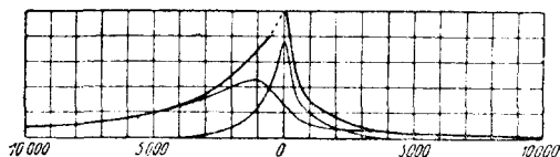
Рис. 3. Распределение пространственных плотностей звезд в большой Галактике по Сирсу. Медленное падение частот в направлении \lambda 325°, быстрое падение в противоположном направлении. Была произведена попытка разложения наблюдаемого распределения (верхняя кривая) на симметричное местное распределение и на асимметричное распределение (две нижних кривых)
