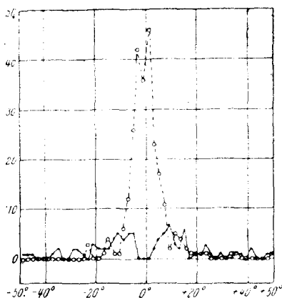
Рис. 5. Распределение рассеянных (белые кружочки) и шарообразных (черные точки) звездных скоплений по галактическим широтам
