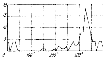
Рис. 6. Распределение шарообразных звездных куч по галактическим долготам
