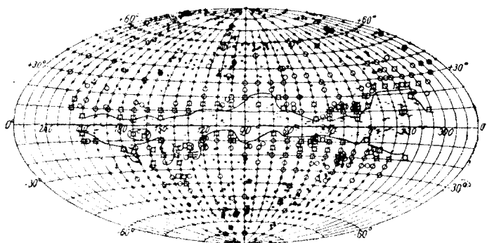
Рис. 8. Распределение на небе внегалактических туманностей
