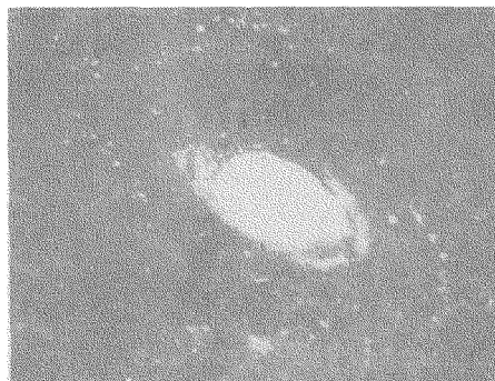
Рис. 7. Спиральная туманность, ветви которой частично кажутся распавшимися на звезды
