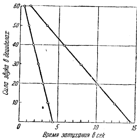
Рис. 3. Спадание силы звука в реверберационной комнате. Частота 500 \pm 50 Hz. Коэффициент поглощения материала 0,85.
