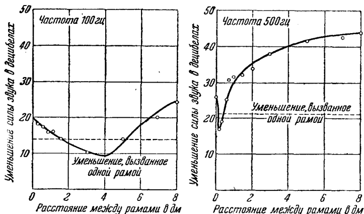
Рис. 4. Влияние расстояния между рамами двойного окна на величину звукоизоляции. Кривые показывают минимум звукоизоляции.
