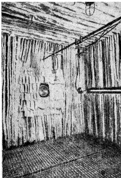
Рис. 6. Заглушенная комната для акустических измерений
