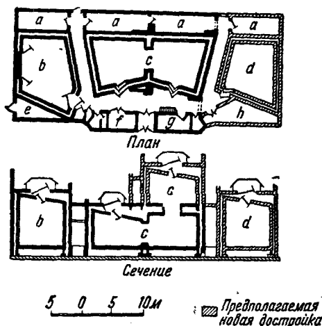
Рис. 1. План акустической лаборатории: a — измерительные комнаты, b — реверберационная комната, c — комната для измерения звукоизоляции, d — заглушенная комната, e — комната воздушного отопления, f — аккумуляторная, g — электротехническая, h — кладовая
