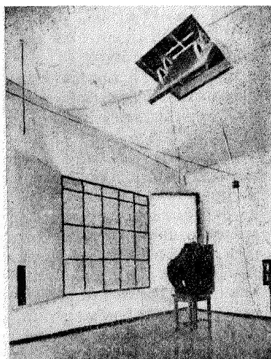
Рис. 2. Реверберационная комната. На фотографии видны: громкоговоритель, микрофон, исследуемая панель из звукопоглощающего материала
