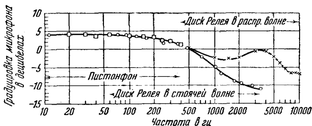
Рис. 7. Кривые градуировки эталонного микрофона.
