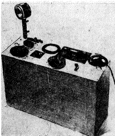
Рис. 8. Переносный акустиметр (шумомер) для объективного измерения силы звука и уровня громкости
