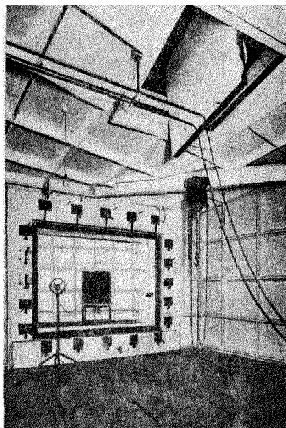
Рис. 5. Камеры для определения звукоизоляции с окном, в которое вставляется исследуемый образец
