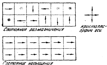
Рис. 8. Элементарные области в монокристалле железа
