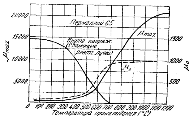
Рис. 19. Возрастание магнитной проницаемости благодаря уменьшению внутренних напряжений посредством прокаливания (Дилингер и Хаурт)
