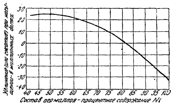
Рис. 16. Магнитострикция насыщения в различных пермаллоях (Мак-Киган и Чюфи, Шульце)
