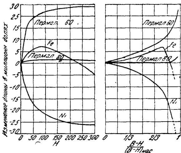
Рис. 15. Магнитострикция в железе, никеле и в двух железоникелевых сплавах (пермаллой)
