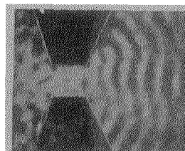
Рис. 10. Ультразвуковая волна, выходящая из щели шириной в 2 длины волны, по Гроссману и Гидеману.
