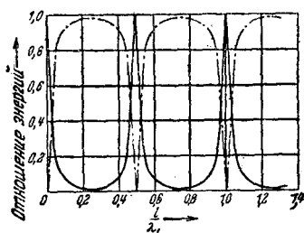
Рис. 13. Зависимость проницаемости и отражательной способности разделяющей стенки от отношения толщины стенки к длине волны, по Бойлю — Раулинсону.
