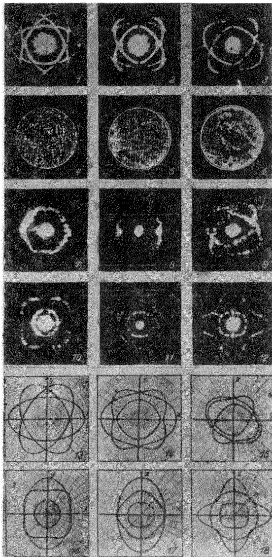
Рис. 14. Интерференционные картины колеблющихся кристаллов, по Шефферу и Бергману: 1—3—кварц, экспериментальные картины, 4—6—сечения решетки кварца (экспериментальные), 7—9—дифракционные явления на сечении кварцевой решетки (экспериментальные), 10—12—барит, экспериментальные кривые, 13—15—кварц, теоретические кривые, 16—18—барит, теоретические кривые.
