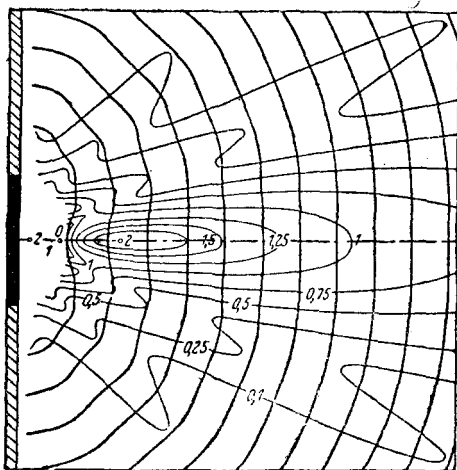
Рис. 9. Волновое поле у круглой поршневой мембраны радиуса 1,75 \lambda , по Гроссману и Гидеману.
