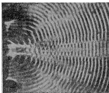
Рис. 12. Звуковое поле перед мембраной, изображенной на рис. 11. при большой интенсивности звука, по Гидеману и Асбаху.
