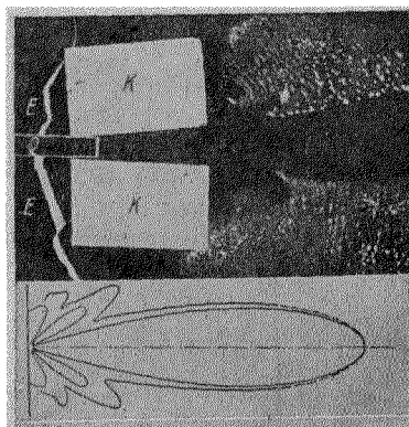
Рис. 8. Пыльная фигура перед щелью шириной 2,65 длины волны; частота — 100 кГц. Внизу для сравнения изображены огибающая поверхности, свободной от песка, и характеристика направленности, по Гроссману и Гидеману.
