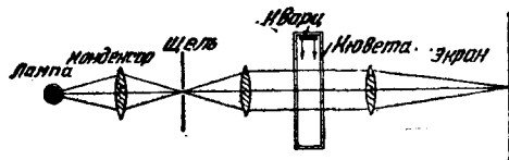
Рис. 2. Схема оптической установки, по Дебаю и Сирсу.
