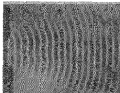
Рис. 11. Звуковое поле перед прямоугольной поршневой мембраной. Ширина кварца 4,85 длины волны, частота 3300 килогерц, по Гидеману и Асбаху.
