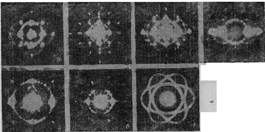
Рис. 6. Интерференционные картины Шеффера—Бергманна. 1—Лауэграмма жидкости, пронизываемой тремя взаимноперпендикулярными звуковыми пучками. 2—Дифракционные картины колеблющегося стеклянного кубика.
