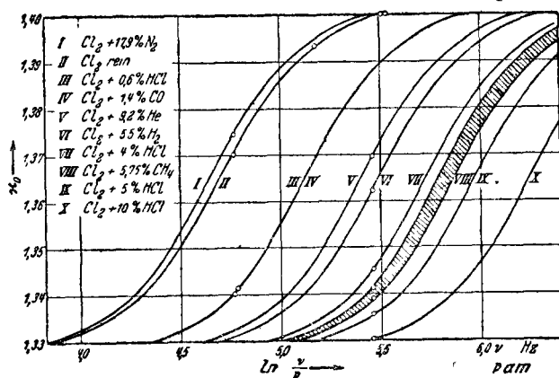
Рис. 18. Дисперсия звука в хлоре с примесями при комнатной температуре, по Эйкену и Беккеру.
