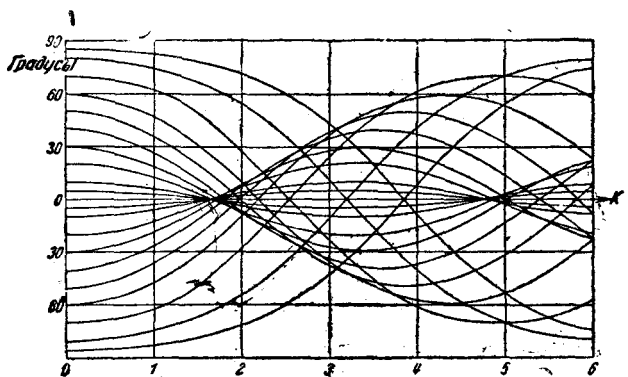
Рис. 3. Ход световых лучей в среде, пронизываемой звуковыми волнами, по Люка и Бикару.
