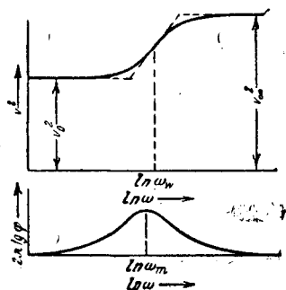
Рис. 16. Дисперсия и поглощение звука в многоатомных газах по Кнезеру.
