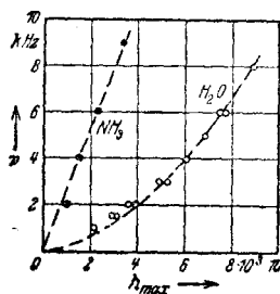
Рис. 17. Частота максимального поглощения в кислороде в зависимости от концентрации загрязняющих газов, по Кнезеру и Кнудсену.
