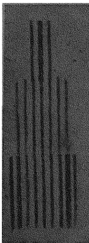
Рис. 4. Зависимость интенсивности дифракционных явлений от интенсивности ультразвука, по Бери.
