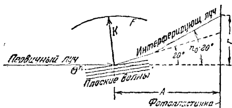
Рис. 15. Возникновение интерференционных фигур, по Фюсу и Людлофу.
