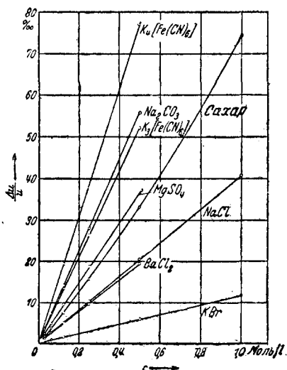
Рис. 19. Зависимость скорости звука от концентрации, по Бахему.
