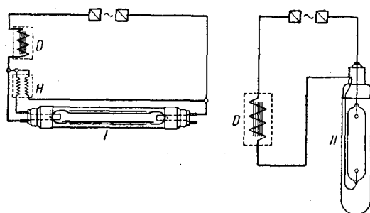
Рис. 12. Включение натровой (I) и ртутной высокого давления (II) ламп.
