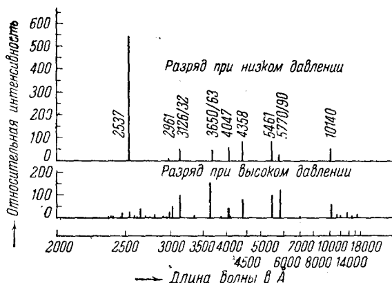
Рис. 14. Распределение энергии в спектре ртутных ламп низкого и высокого давления при одинаковом полном излучении.
