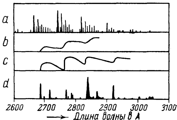
Рис. 7. Спектр флуоресценции бензола при возбуждении ультрафиолетовыми линиями ртути: а) газообразный бензол, б) жидкий, в) твердый при 0° С, д) твердый при -180° С.
