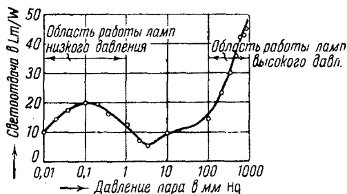
Рис. 13. Светотдача разряда в парах ртути в зависимости от давления пара.
