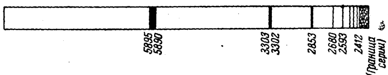
Рис. 4. Резонансная серия натрия
