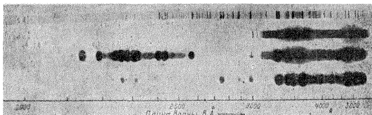
Рис. 9. Флуоресценция вольфрамата кальция с и сернистого цинка d , a — непосредственная фотография возбужденного спектра, b — фотография того же спектра после фильтрации через прозрачную стеклянную пластинку.
