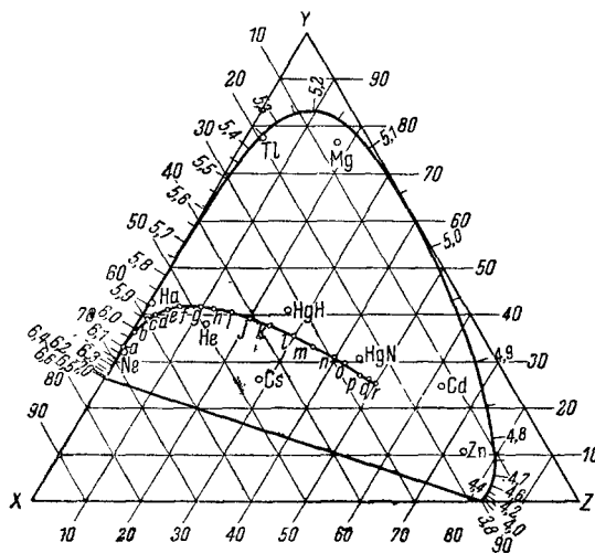
Рис. 3. Максвелл-гельмгольцевский цветовой треугольник.
