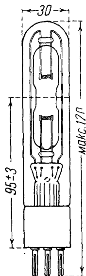
Рис. 15. Натриевая спектральная лампа для переменного тока.
