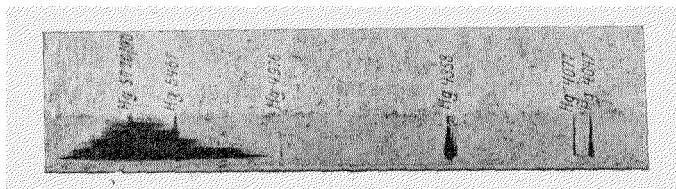
Рис. 10. Спектр ртутной лампы, использующей флуоресценцию. Снято с помощью ступенчатого фильтра.
