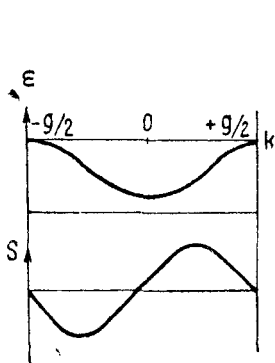
Рис. 3. Зависимость энергии и тока от волнового числа. Сильно связанные электроны (одномерная задача)
