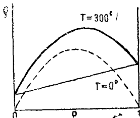
Рис. 12. Изменение кривой сопротивления при повышении температуры смеси.
