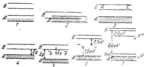
Рис. 3. Схемы энергетических уровней в металлах, полупроводниках и изоляторах.
