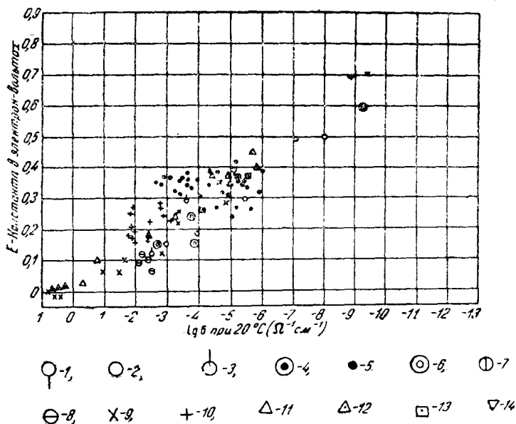
Рис. 1. Связь между константой E \left( \sigma = ae^{-\frac{Ee}{kT}} \right) и удельной электропроводностью \sigma .
