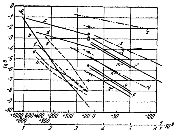
Рис. 2. Температурная зависимость удельной электропроводности \text{SiO}_2
