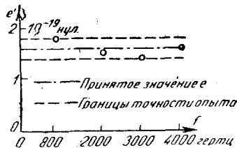
Рис. 9. Частотная зависимость дробового эффекта в фотоэлементе (Орбан) — — — принятое значение e ; — — — границы точности опыта.
