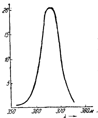
Рис. 6. Пример частной характеристики усилителя Хелла и Уильямса.
