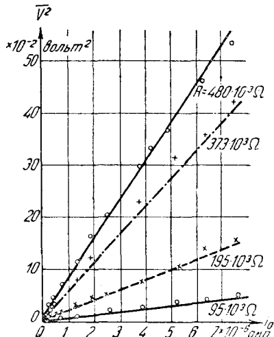
Рис. 8. Зависимость дробового эффекта в фотоэлементе от силы фототока (Орбан).
