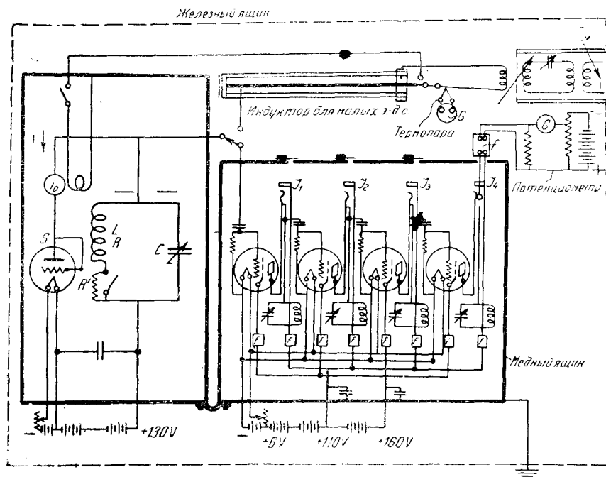
Рис. 5. Схема установки Хелла и Уильямса. 1
