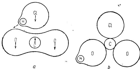
Рис. 2. a —движение атомов при столкновении молекул \text{HCl} и \text{CO}_2 ; b —молекула \text{SiCOOH} (по Эйкену и Беккеру).
