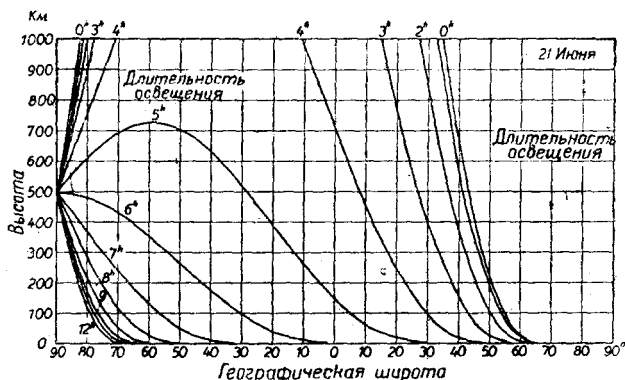
Рис. 1. Солнечный восход в свободной атмосфере вдоль меридиана. Линии соединяют точки, в которых солнце восходит в определенный час.
