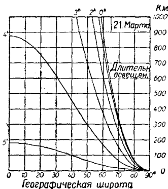
Рис. 2. То же, что и рис. 1.
