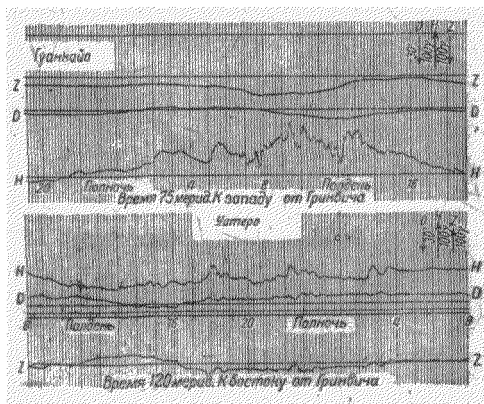
Рис. 24б. Регистрации тех же обсерваторий в возмущенный день с интернациональным характеристическим числом 1,6 (4 декабря 1929).
