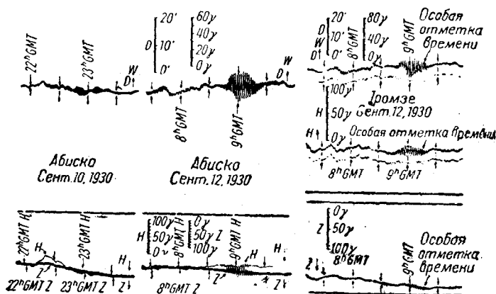
Рис. 23. Микропульсации склонения D , горизонтальной интенсивности H , и вертикальной интенсивности Z по регистрациям в Абиско (Швеция) и Тромсё. Время — среднее Гринвичское.
