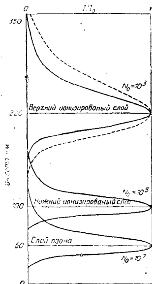
Рис. 42. Схема трех атмосферных слоев, в которых поглощается отвесно падающее солнечное излучение. N_0 есть максимальное число диссоциировавших молекул и ионизированных атомов в 1 \text{ см}^3 в 1 сек. (по Чэпману).
