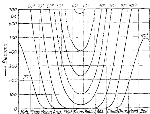
Рис. 5. Высота границы солнечной тени в полночь на широтах 40—90° в течение года.
