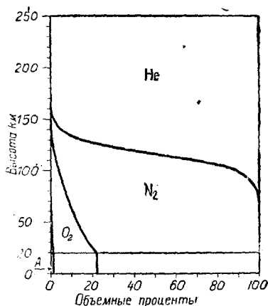
Рис. 9. Процентный состав атмосферы в тех же предположениях, что и на рис. 8, но без водорода.
