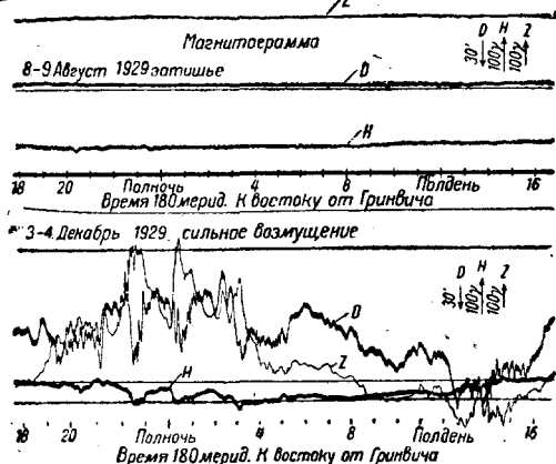
Рис. 25. Регистрации станции в южной полярной области на южн. широте 78,6° (те же дни, что на рис. 24а и б).
