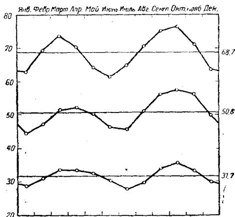
Рис. 35. Годовой ход магнитной активности Земли в сильно возмущенный год (сверху), в слабо возмущенный (в середине) и в год затихья (внизу).
