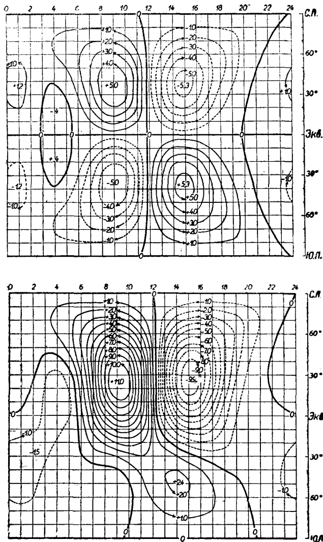
Рис. 18 и 19. Карты атмосферной системы тока, вычисленные из лунных вариаций земного магнетизма к моменту новолуния. Рис. 18 — годовое среднее, рис. 19 — северное лето. Меридианы обозначены местным лунным временем, которое к моменту новолуния достаточно точно совпадает с солнечным временем (12 = полдень), так что дневная сторона Земли занимает среднюю часть карты. Значения функции тока в единицах 1000 А; между каждыми двумя линиями течет 500 А в направлении стрелки.
