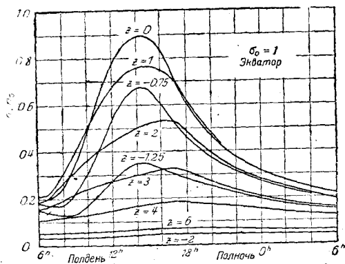
Рис. 38. Дневной ход числа ионов в 1 \text{ см}^3 , в долях того максимального числа ионов n_0 , которое устанавливается при достаточно длительном отсвесе подающим излучении на высоте максимальной ионизации; числа даны для различных высот над экватором при двух различных предположениях относительно константы \sigma_0 (по Чэпману).
