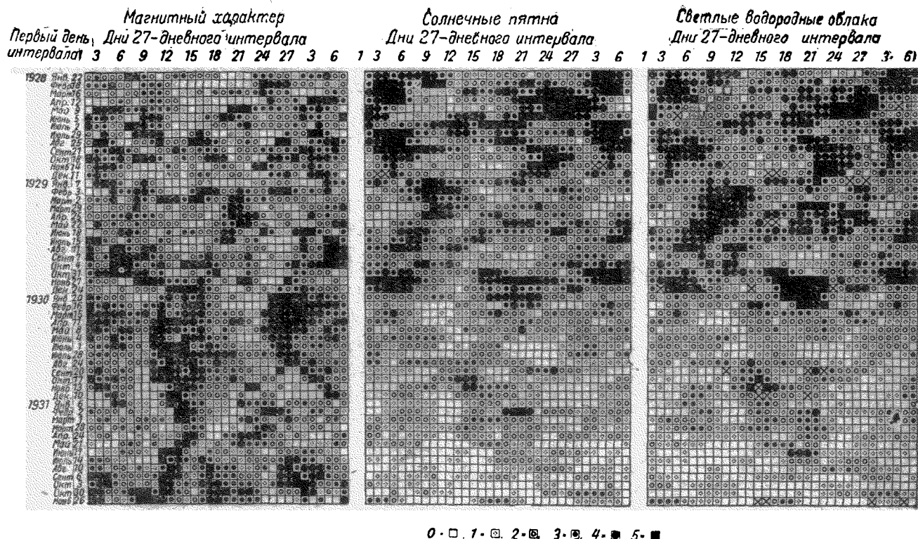
Рис. 29. Демонстрация периода обращения Солнца в значениях магнитной активности Земли (слева), в относительных числах солнечных пятен (середина), и в интенсивности светлых водородных облаков в центральной части солнечного диска (справа). Шкала: 0 — спокойно, 5 — сильно возмущено, или много пятен или облаков. В правой части некоторые дни без наблюдений помечены крестом.
