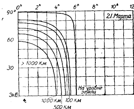
Рис. 3 и 4. Карты полушария между полуночным и полуденным меридианами. Меридианы обозначены их истинным местным временем. Линии соединяют точки солнечного восхода на поверхности Земли, на высоте 50, 100, 250, 500 и 1000 км.
