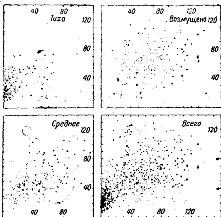
Рис. 34. Одновременные месячные средние относительных чисел солнечных пятен (абсцисса) и магнитной активности Земли (ордината) за годы 1872—1930. Слева наверху: 20 лет низкой активности, слева внизу: 19 лет средней активности, справа наверху: 20 лет высокой активности, справа внизу: все 708 месячных средних. Коэффициенты корреляции в том же порядке: +0,30 ; +0,36 ; +0,38 ; +0,65 .
