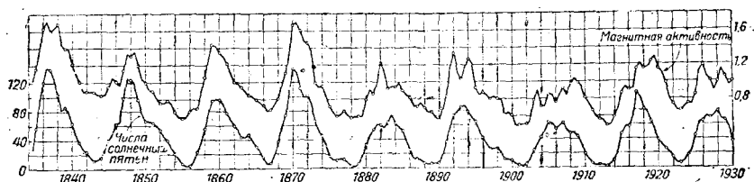
Рис. 31. Годовое среднее магнитной активности Земли (вверху) и относительных чисел солнечных пятен за годы 1835—1930. Обычные годовые средние отмечены маленькими кружками.
