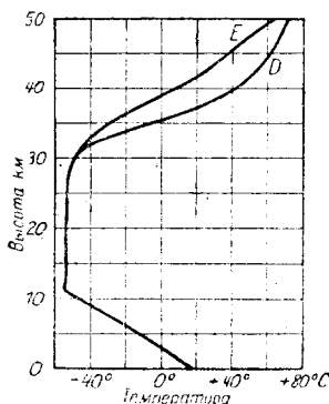
Рис. 7. Температура верхней стратосферы по наблюдениям над распространением звука. E — английские данные (по Уипплу), D — немецкие (по Дуккерту).
