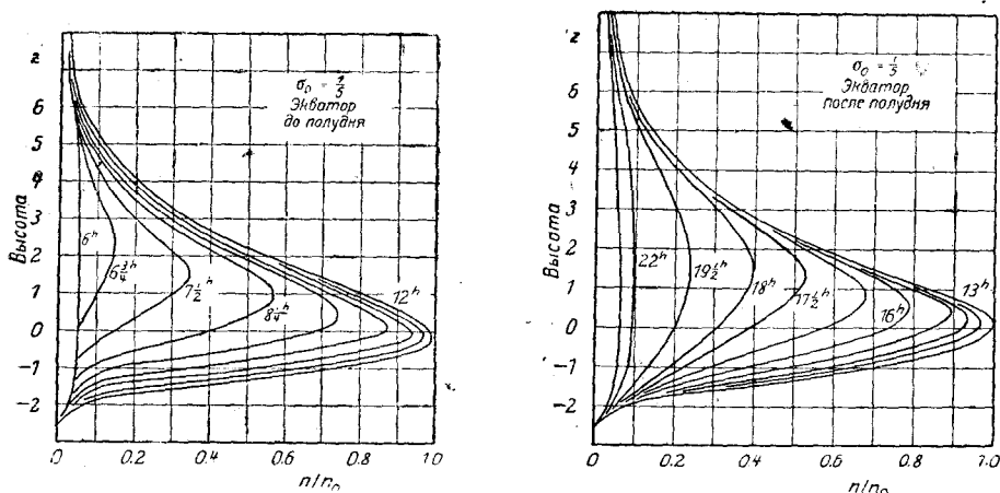
Рис. 40. Распределение числа ионов в зависимости от высоты в различное время дня (по Чепману).
