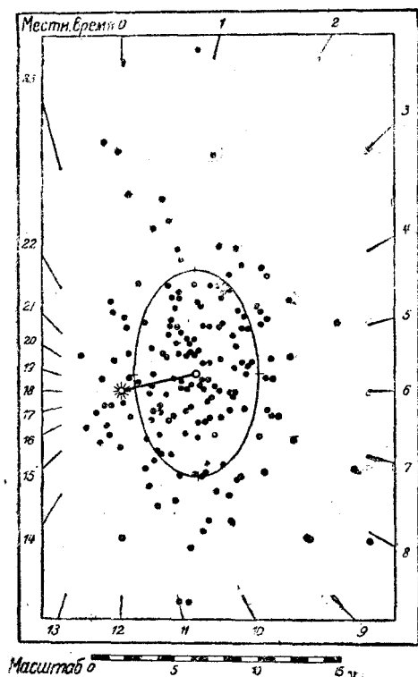
Рис. 21. Часовая шкала для 24-часовой синусоидальной волны суточно-периодических вариаций горизонтальной интенсивности за 171 день затишья (обсерватории Уотеро, Зап. Австралия). Начальная точка координатной системы обозначена звездочкой.
