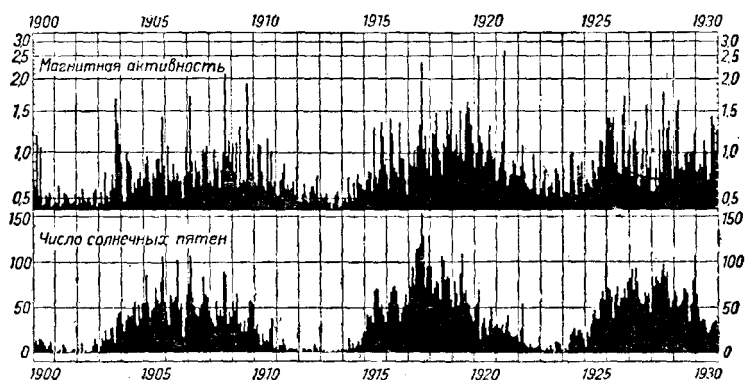
Рис. 32. Месячное среднее магнитной активности Земли (вверху) и относительных чисел солнечных пятен (внизу) за годы 1900—1930.
