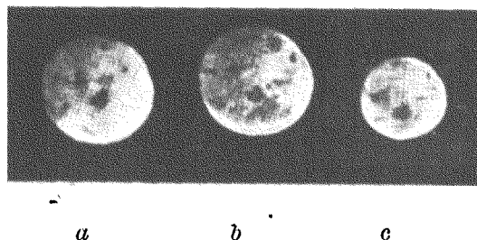
Рис. 19. Образование облака пространственного заряда у поверхности толстого оксидного слоя. a —пространственный заряд отсутствует; b —увеличение излучающего островка пространственным зарядом при увеличении накала катода, c —восстановление резкого изображения излучающего островка путем изменения фокусного расстояния электроно-оптической системы.
