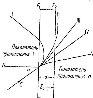
Рис. 5. Пути электронов в двойном электрическом слое.
