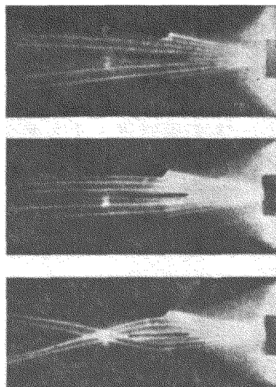
Рис. 7. Демонстрационная электростатическая линза Брюхе-Йогансона.
