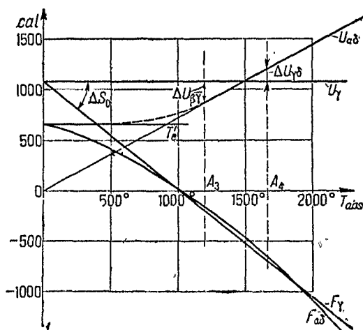
Рис. 4. Общая и свободная энергия центрированного и центрированного железа (имеет силу лишь выше точки Кюри).
