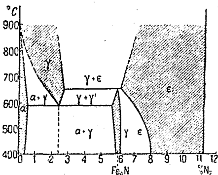
Рис. 16. Диаграмма состояния железо-азот по Эйзенгунту и Кауппу. 83
