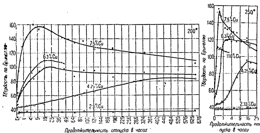
Рис. 21, а и б. Ход твердости при выделении меди из пересыщенных твердых растворов с серебром по Агееву, Ганзену и Заксу. 40 (Температуры отпуска 200° и 250°.)
