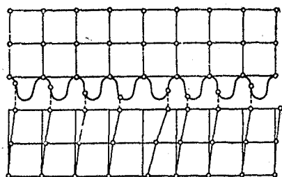
Рис. 23. Механически устойчивое сцепление пластинок скольжения.
