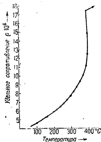
Рис. 6. Сопротивление \text{AuCu} в термодинамическом равновесии (по Грубе).
