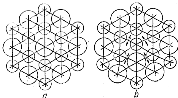
a — сетчатые плоскости \text{AuCu}_3 с упорядоченным атомным распределением; b — малые искажения распределения благодаря замещению атомных пар.
