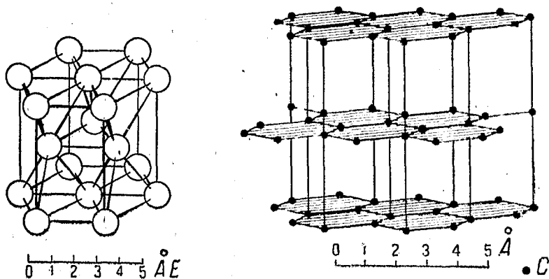
Рис. 1. Структура магния (гекс. 12) и графита как примеры координационной и слоистой решеток.
