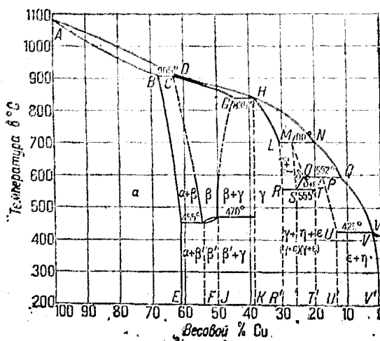
Рис. 15. Диаграмма состояния медь-цинк по Бауэру и Ганзену (из Зауервальда (Sauerwald, Metallkunde, S. 414)).
