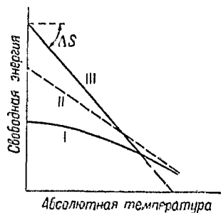
I — правильное расположение, II — неправильное расположение, III — неправильное расположение с увеличенной электронной энтропией.
