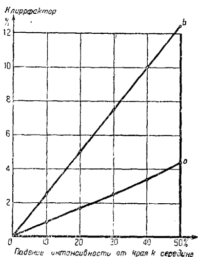
Рис. 80. Клирфактор при воспроизведении фонограммы типа переменной ширины с неоднородно освещенной щелью.
