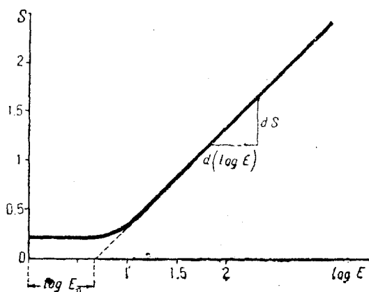
Рис. 75. Характеристическая кривая.
