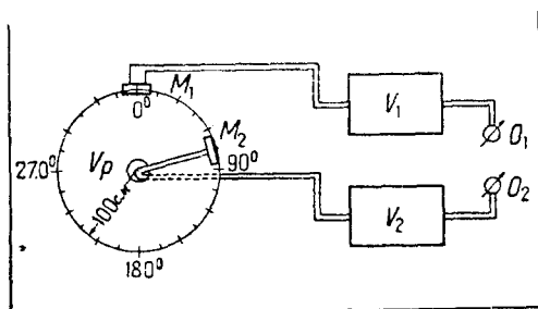
Рис. 47. Схема исследований направленности человеческого голоса.
