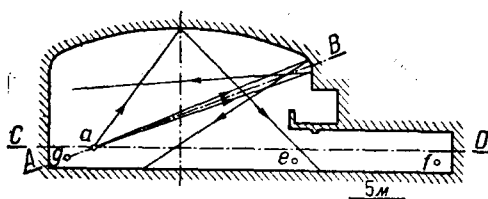
Рис. 55. Продольное сечение актового зала Фрейбургского университета.
