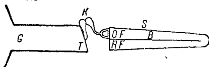
Рис. 39. G — слуховой проход, K — слуховые косточки; T — барабанная перепонка; OF — овальное окно; S — улитка с основной мембраной B (схематические).
