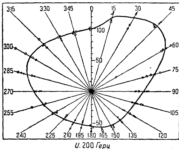
Рис. 48а. Направленное действие голоса при U .
