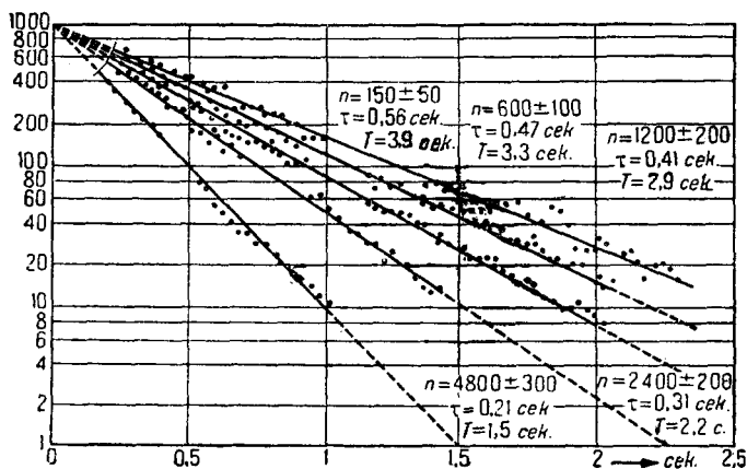
Рис. 63. Измерения поглощения звука различными людьми (по Мейеру).
