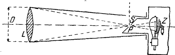
Рис. 25. Приемник оптической телефонии с фотоэлементом по Циклеру 72 .
