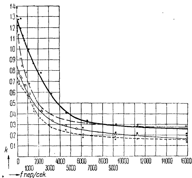
Рис. 15. Зависимость от частоты относительных колебаний света дуги по Яуману 21 .
