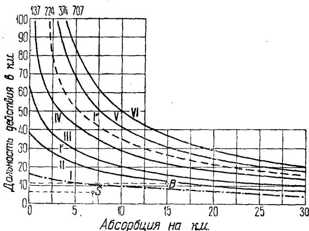
Рис. 6. Зависимость дальности действия от абсорбции при различной интенсивности передачи по Циклеру (цифровые данные см. таблицу).
