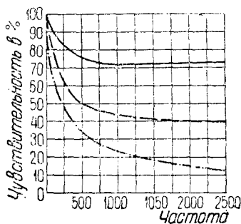
Рис. 4. Зависимость чувствительности различных элементов от частоты:
