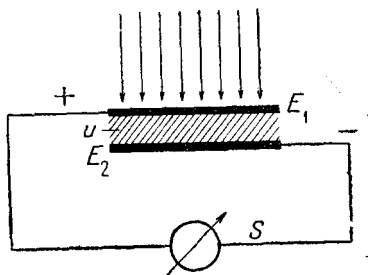
Рис. 1. Схема фотоэлемента по Ланге 22
