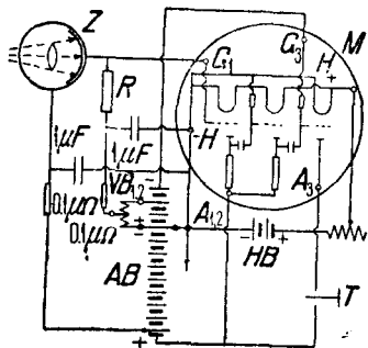
Рис. 26. Приемник оптической телефонии с фотоэлементом по Циклеру. Электрическая часть.
