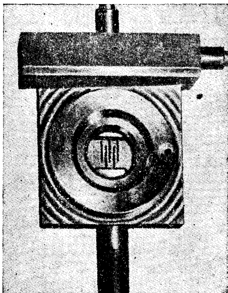
Рис. 21. Керровский конденсатор большой мощности по Ильбергу 20 .
