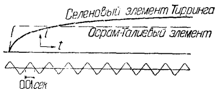
Рис. 3. Кривая тока при внезапном освещении по Зевигу 58 .
