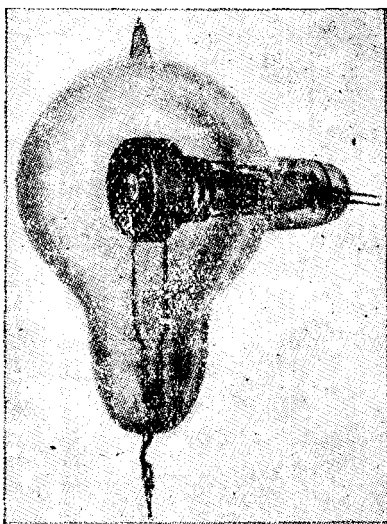
Рис. 18. Лампа тлеющего разряда по Пирани 55 .
