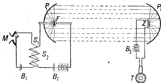
Рис. 10. Оптический телефон по Сймону 59 . F — дуга, M — микрофон, S_1, S_2 — трансформатор, P — параболическое зеркало, Z — селеновый элемент, T — телефон.
