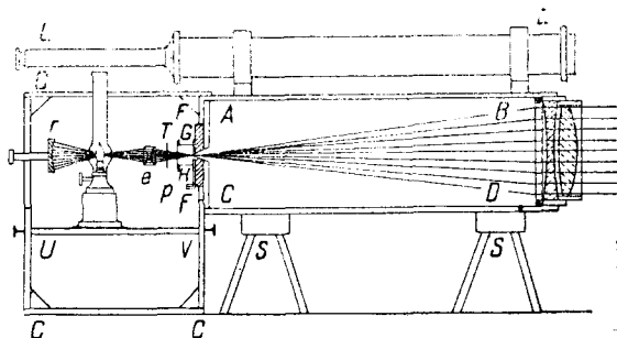
Рис. 9. Оптический телеграф по Манжену 31 .
