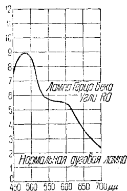
Рис. 11. Спектральное распределение плотности освещения угольной лампы Герца-Бека по отношению к нормальной угольной лампе по Циклеру.
