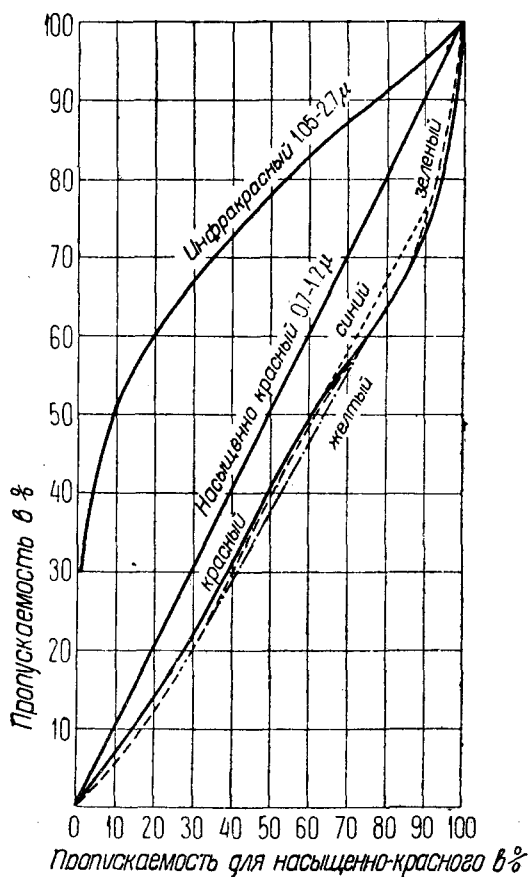
Рис. 8. Пропускательность облака из больших частиц по Андерсону 1.
