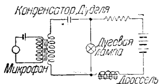
Рис. 13. Схема говорящей дуги по Дуделю 10 .
