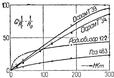
Рис. 5. Связь между фототоком и освещением по Зевигу 58 .
