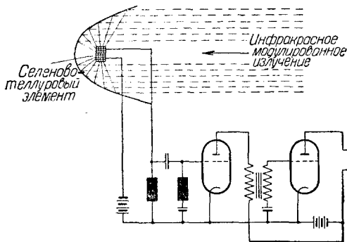
Рис. 27. Приемник ультрафиолетовой телефонии по Шрето 53 .
