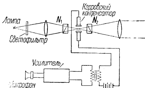
Рис. 20. Модуляция при помощи керровского конденсатора по Шретеру 53 .
