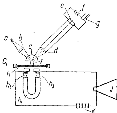
Рис. 22. Схема оптической телефонии по Цейссу 69 для отраженного света.
