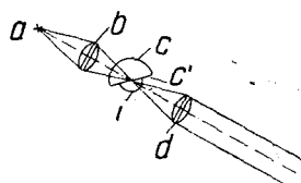
Рис. 23. Ход лучей в схеме Цейсса для проходящего света.
