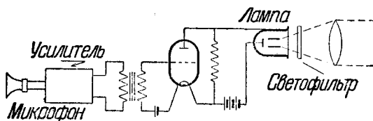
Рис. 19. Модуляция гелиевой лампы по Шретеру 53 .
