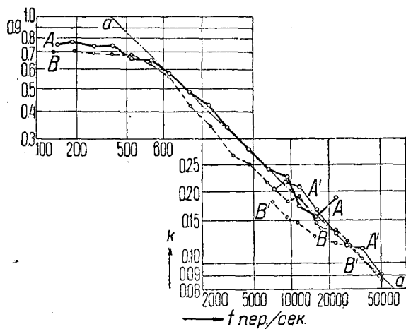
Рис. 16. Зависимость от частоты относительных колебаний света (логарифмический масштаб) по Яуману.
