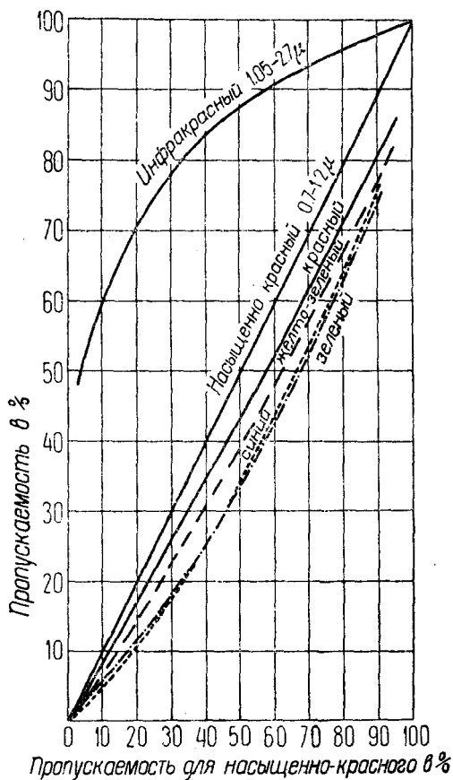
Рис. 7. Пропускаемость облака из малых частиц по Андерсону 1 .
