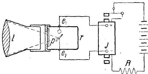
Рис. 24. Приемное устройство для ультрафиолетовой телеграфии по Циклеру 70 .
