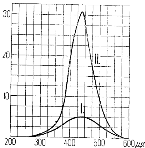
Рис. 12. Спектральное распределение чувствительности калиевого фотоэлемента Пресслера по Циклеру: I — вакуумный элемент, II — газополный элемент.
