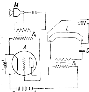
Рис. 17. Расположение для модуляции ртутной лампы по Майорана 26 .
