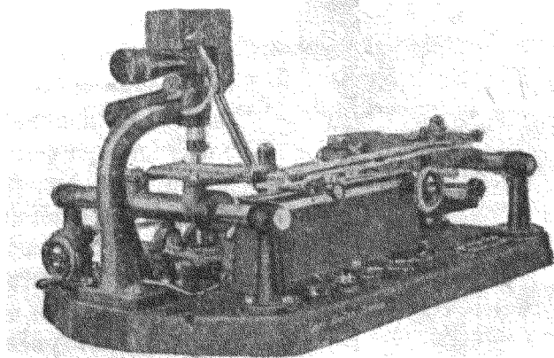
Рис. 12. Микрофотометр Цейса.
