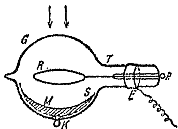
Рис. 1. Схема фотоэлемента.
