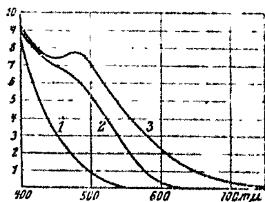
Рис. 8. Кривые спектральной чувствительности Тунгстена-Нава фотоэлементов.
