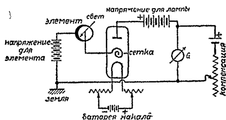
Рис. 14. Усилительная схема по Розенбергу.
