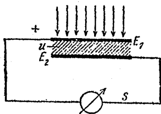
Рис. 9. Схема купроксидного фотоэлемента.
