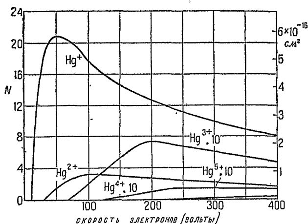
Рис. 1. Число \text{Hg}^+ , \text{Hg}^{2+} , \text{Hg}^{3+} , \text{Hg}^{4+} , \text{Hg}^{5+} ионов на см пути и мм давления при 0°. Справа даны площади эффективного сечения для ионизации атома Hg.
