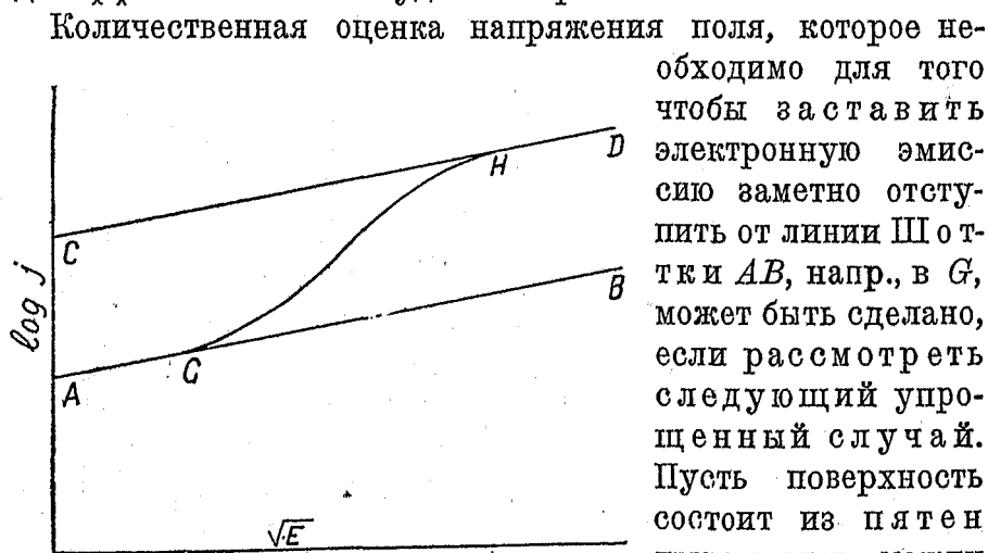
Рис. 4. Влияние размеров „пятна“ на электронную эмиссию.
