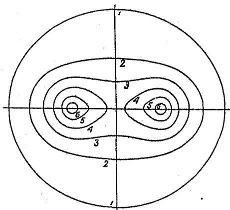
Рис. 6. Распределение плотности при гомеоплярной связи.
