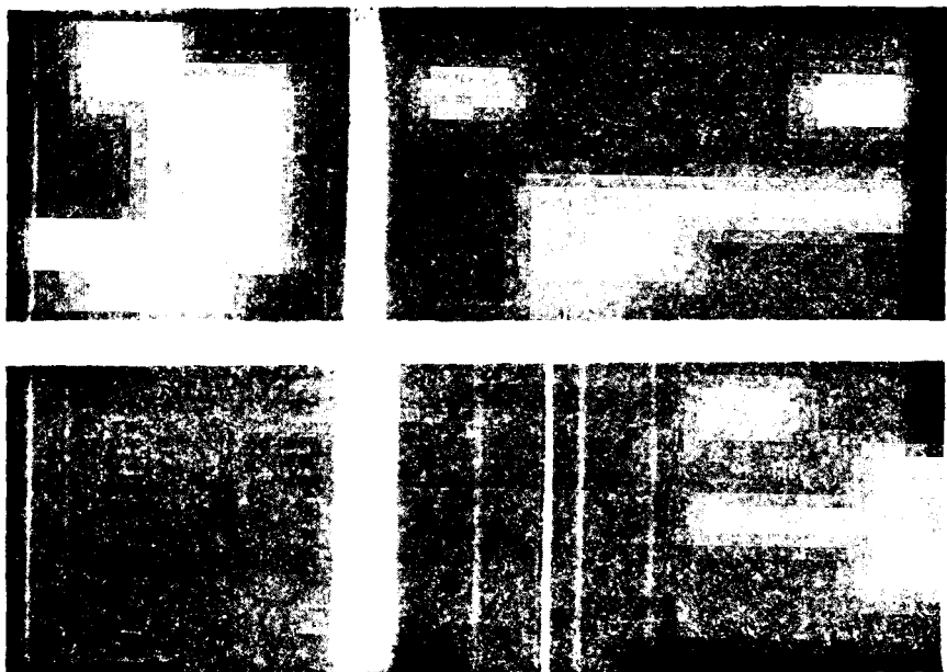
Рис. 4. Спектрограмма света, рассеянного бензолом. Вверху спектр сравнения.
