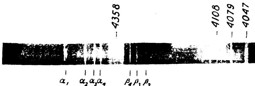
Рис. 5. Спектр рассеяния в \text{CCl}_4 (по Вуду). \alpha_1, \alpha_2, \alpha_3, \alpha_4 — красные трабанты при линии 4358 Å; \beta_1, \beta_2, \beta_3 — соответственные фиолетовые трабанты.
